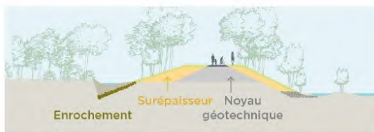
Après – Nouvelle digue
