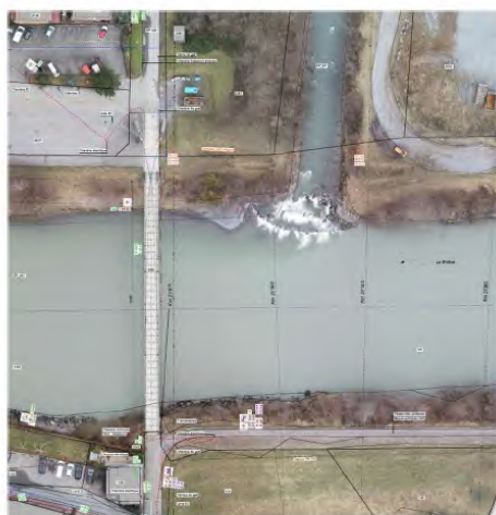
Actuel Passerelle mobilité douce Longueur : 70 mètres Largeur : 3.6 mètres
