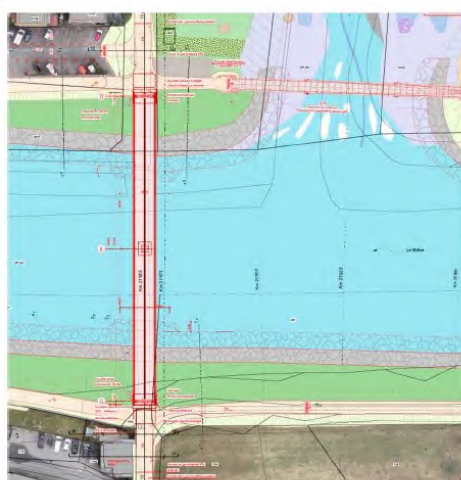
Futur Pont mobilité douce et transport public Longueur : 95 mètres Largeur : 6 mètres
