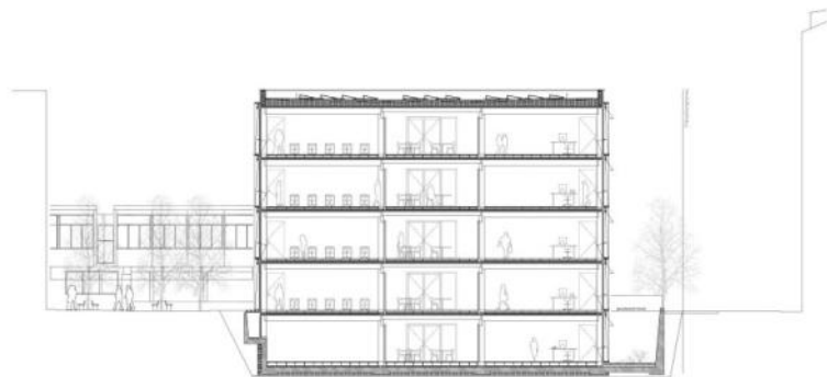
Schnitt A-A
