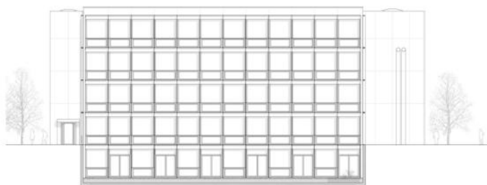
Südfassade
