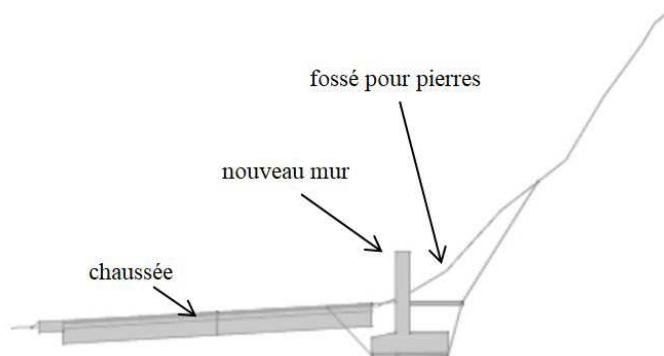
Figure 6 : Mur amont à semelle arrière et fossé de réception des chutes de pierres
