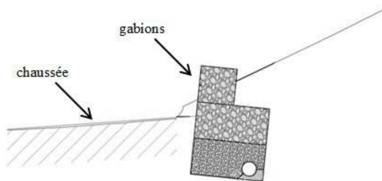
Figure 19 : Mur de soutènement en gabions, coupe-type
