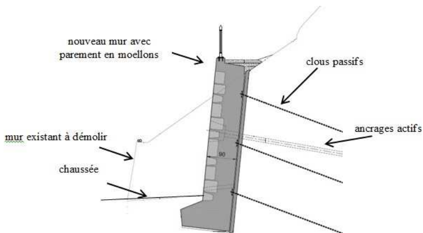
Figure 17 : Mur de soutènement en béton armé, parement en maçonnerie et tirants actifs
