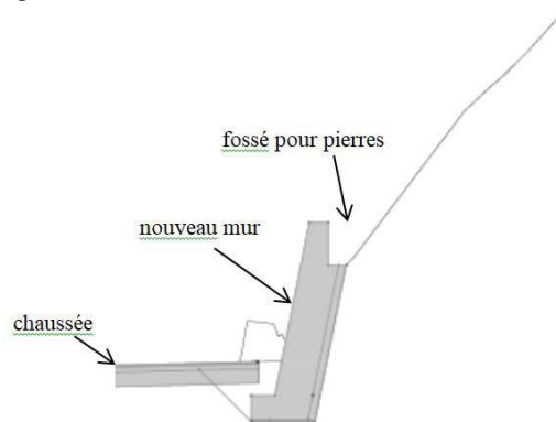
Figure 4 : Mur poids amont avec couronnement pour la réception des chutes de pierres
