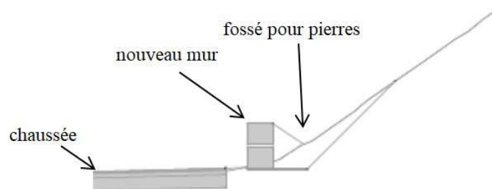
Figure 5 : Mur poids amont en blocs de béton et fossé de réception des chutes de pierres
