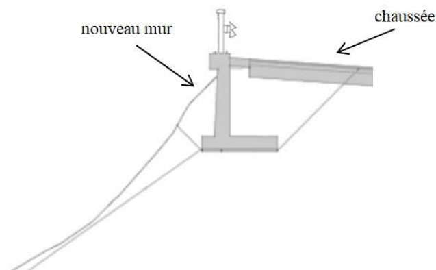
Figure 7 : Mur aval à semelle arrière
