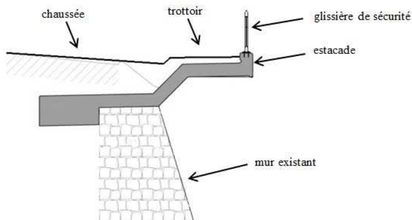
Figure 15 : Estacade sur le ruisseau de Brent, coupe-type sur le mur existant en maçonnerie
