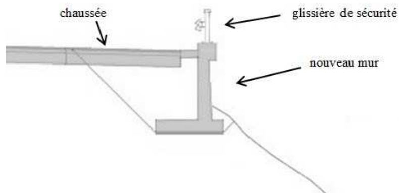
Figure 12 : Mur à semelle arrière, longueurs 22 m et 16 m de part et d'autre du mur poids central
