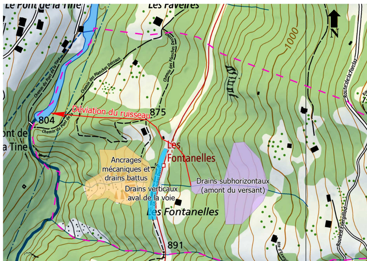
Figure 4 : Représentation schématique du concept prévu de mesures d'assainissement.
