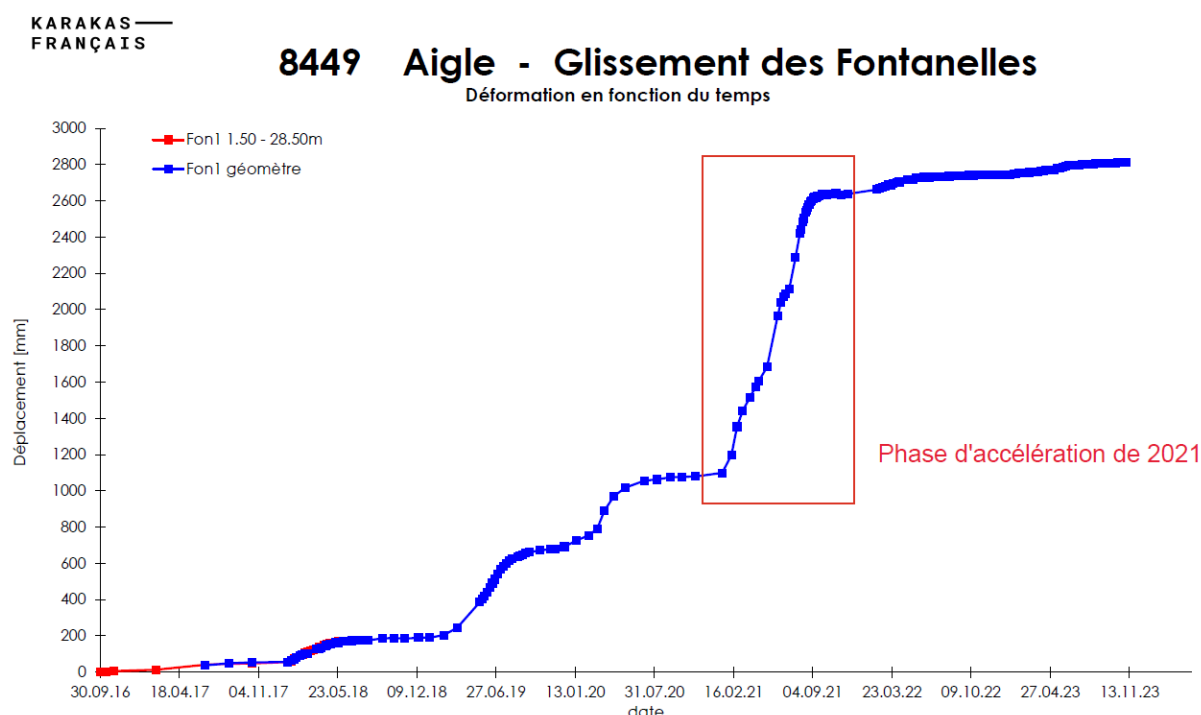
Figure 3 : Suivi des vitesses du glissement au cours du temps. Tiré de (1).
