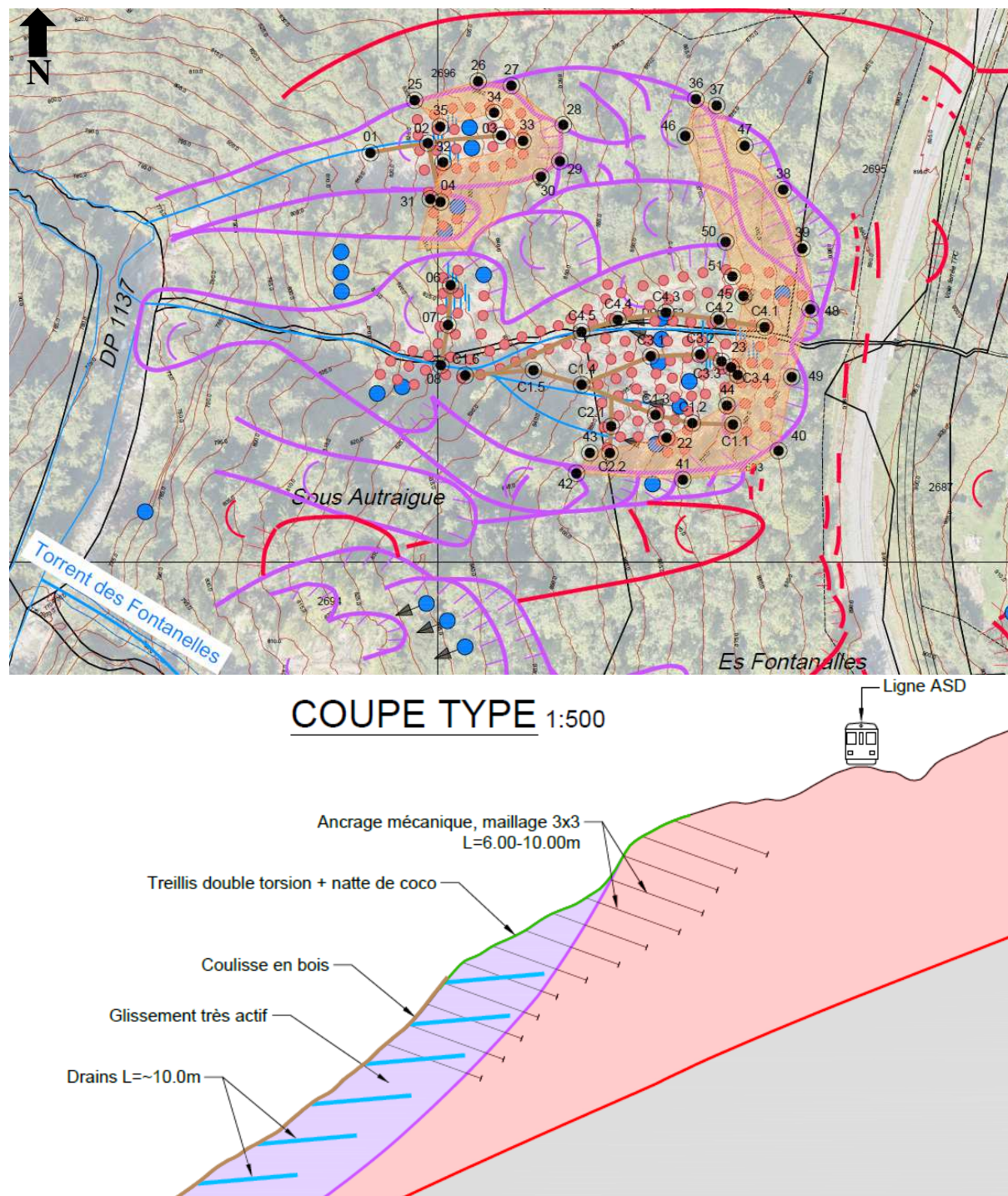
Figure 8 : Plan et coupe-type des ancrages et drains pour éviter la régression de la niche d'arrachement. Tiré de (1).
