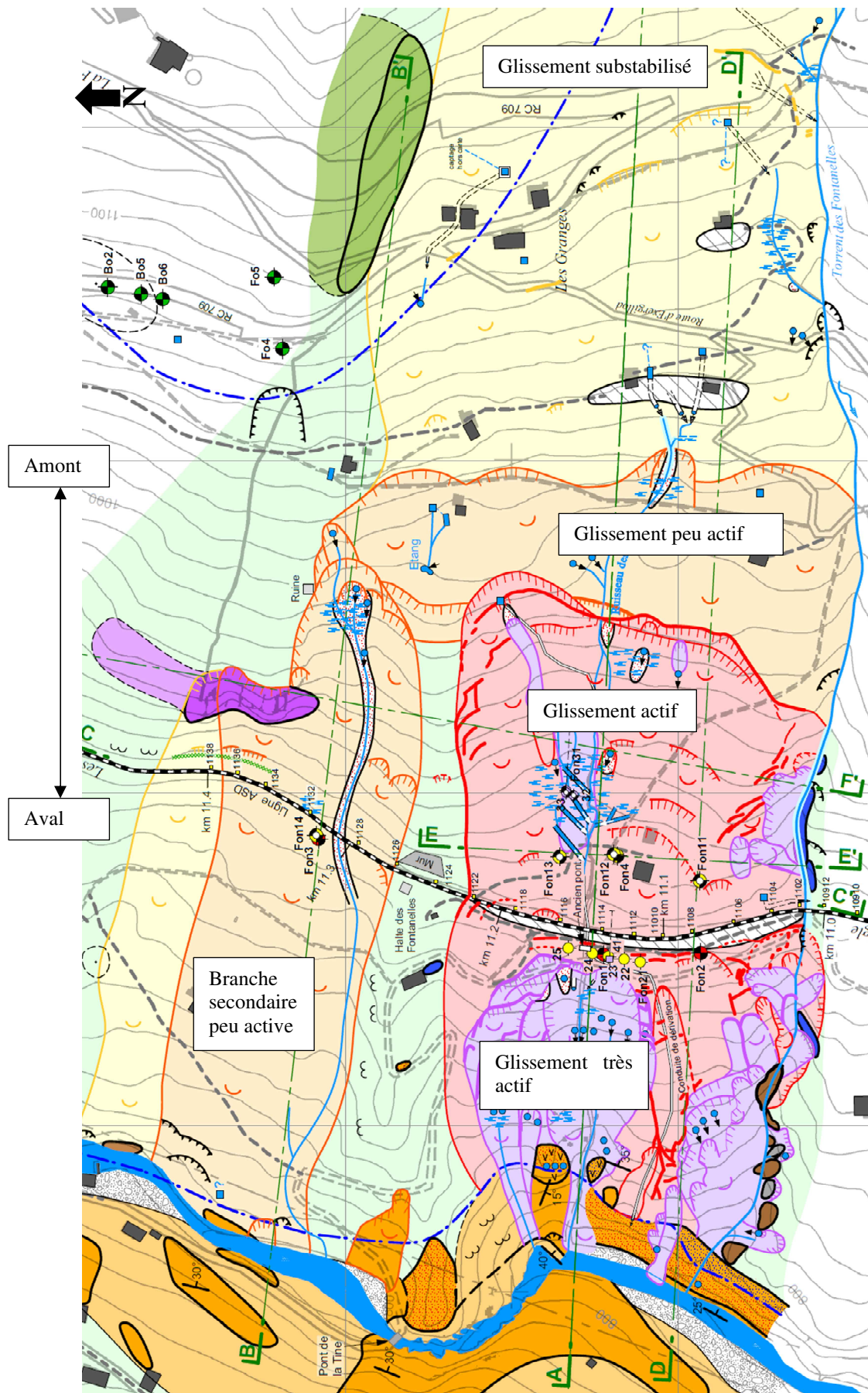
Figure 2 : Carte géologique du glissement des Fontanelles. Tiré de (1).
