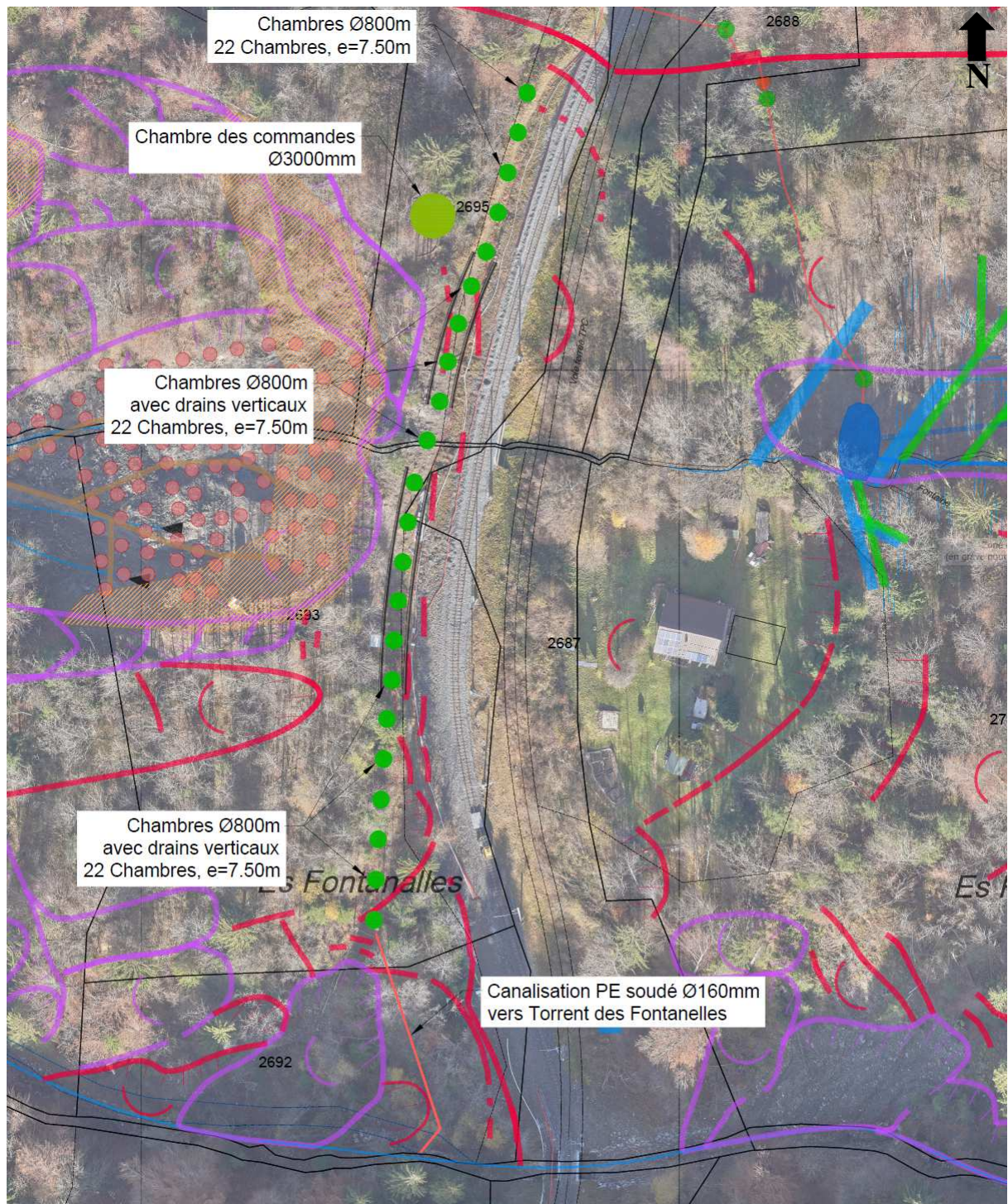
Figure 6 : Plan des drains verticaux (aval de la voie). Tiré de (1).
