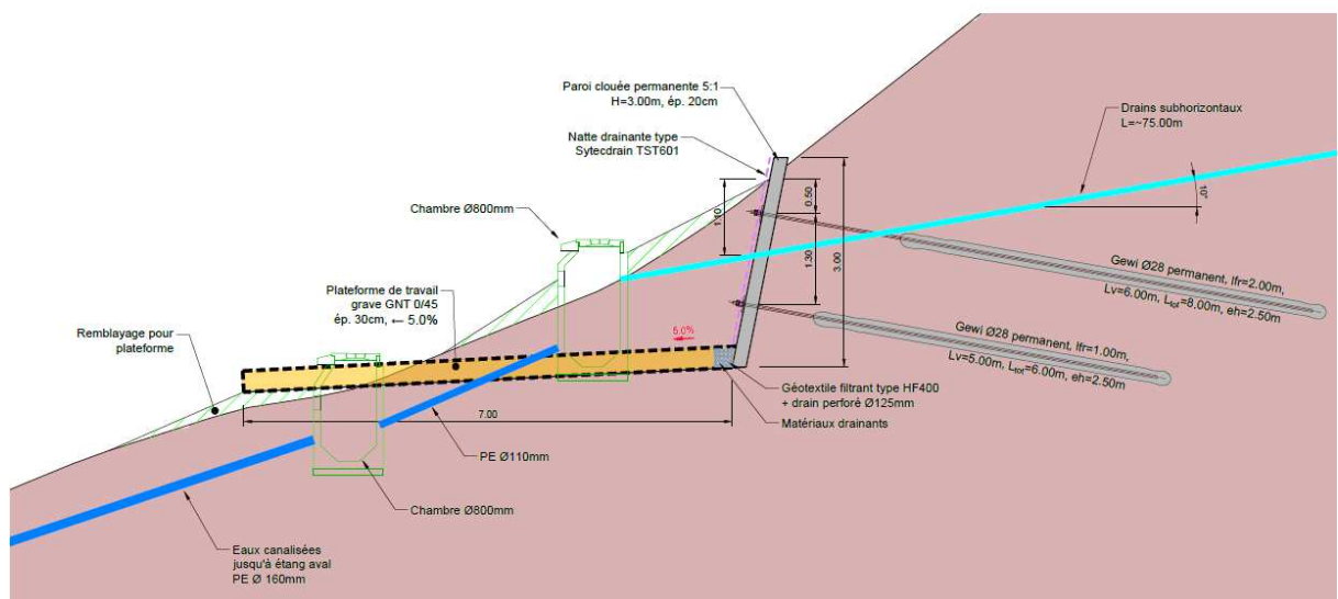
Figure 5 : Plan et coupe-type des drains subhorizontaux (drainage du versant amont). Tiré de (1).
