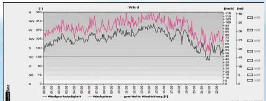
Abb. 4: Gemittelte Windstärken und Böenspitzen für den 29. November 2009, registriert an der Wetterstation Isleten.
