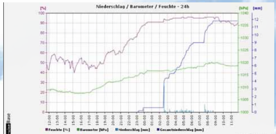
Abb. 3: Verlauf der Messwerte für Feuchte, Luftdruck und Niederschlag am Beispiel des 19. Novembers 2009 (Wechsel von Föhn- zu Nordstaulage?)
