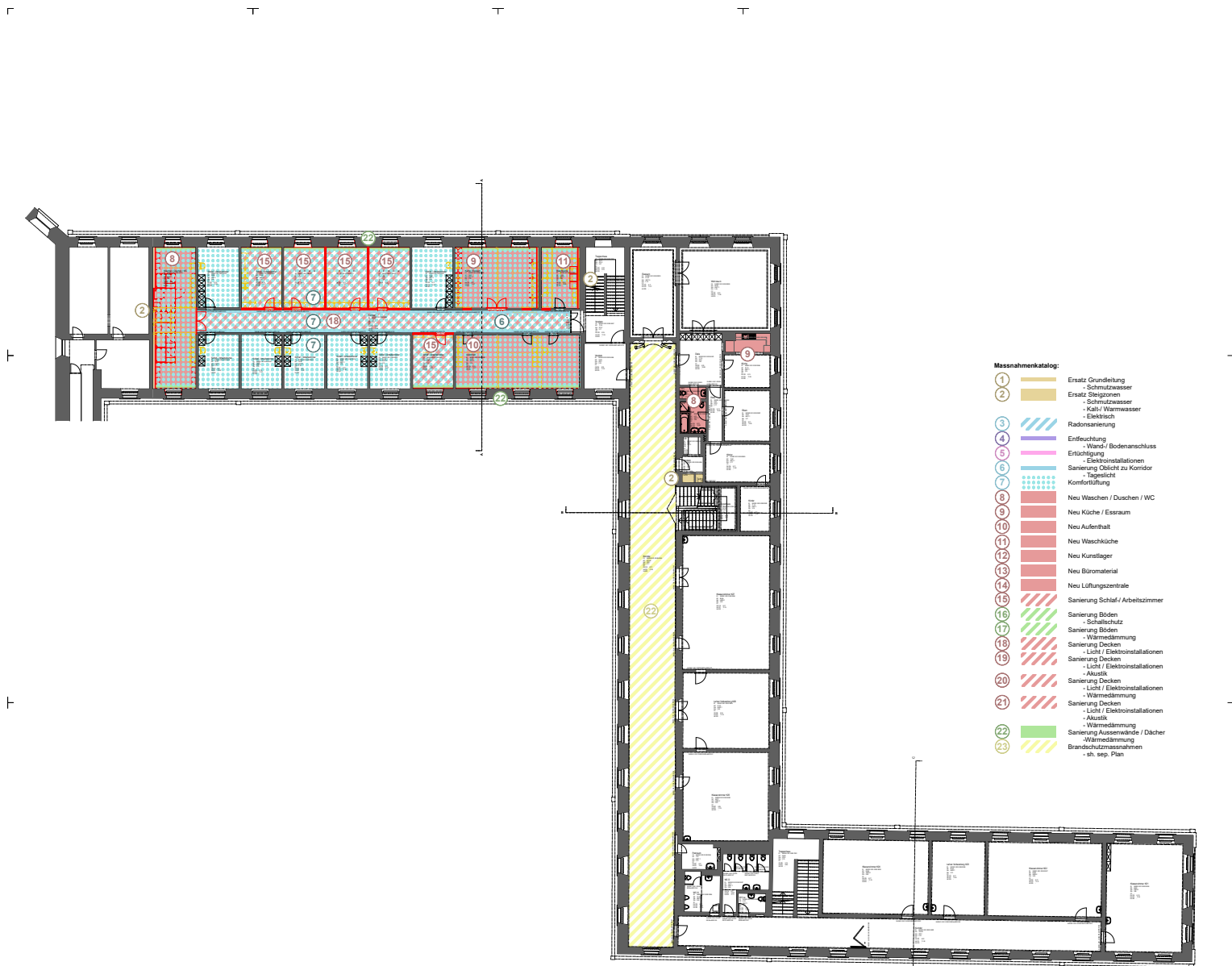
Grundriss 2. Obergeschoss
