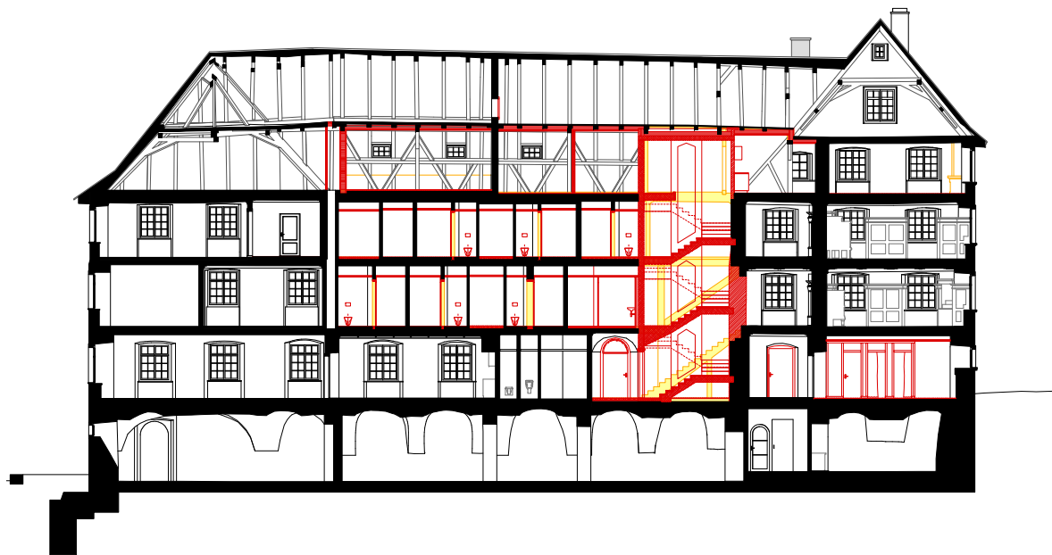
Schnitt C-C
