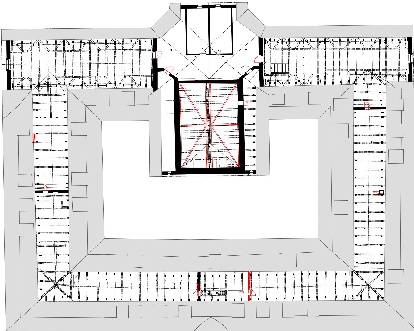
Grundriss Dachgeschoss
