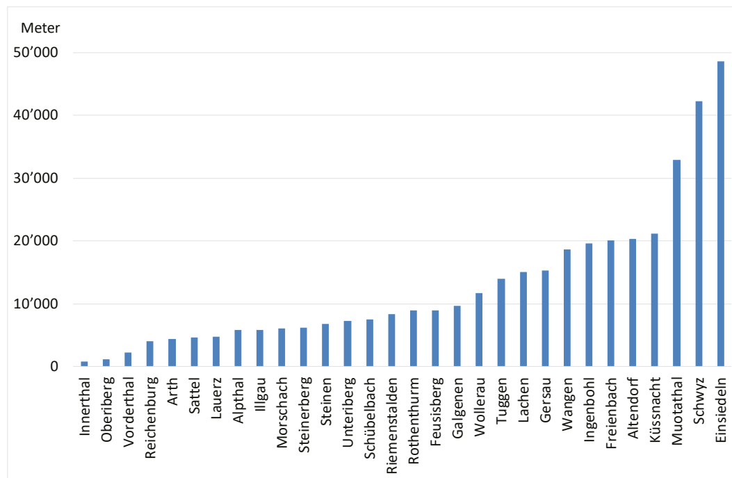
Abbildung 16 Strassenlänge
