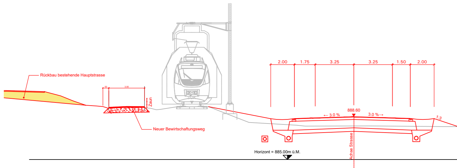
Schnitt 4-4
