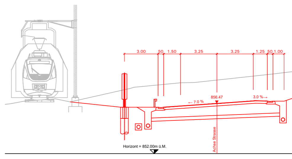
Schnitt 5-5
