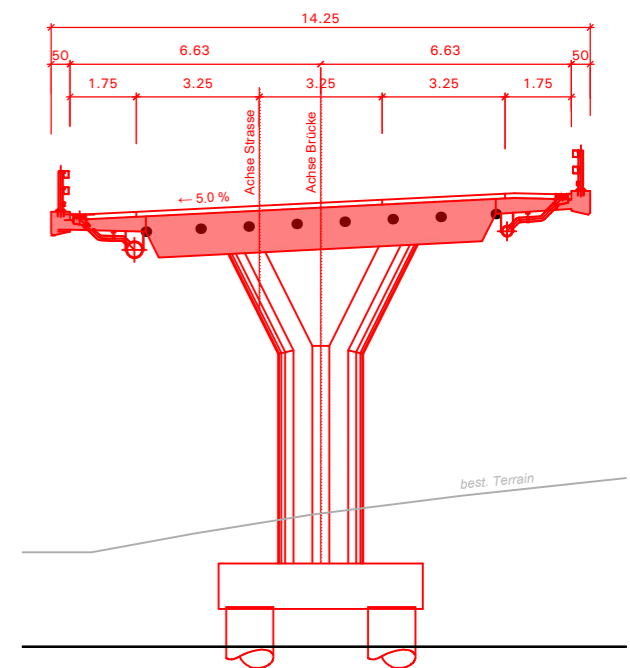
Schnitt 6-6
