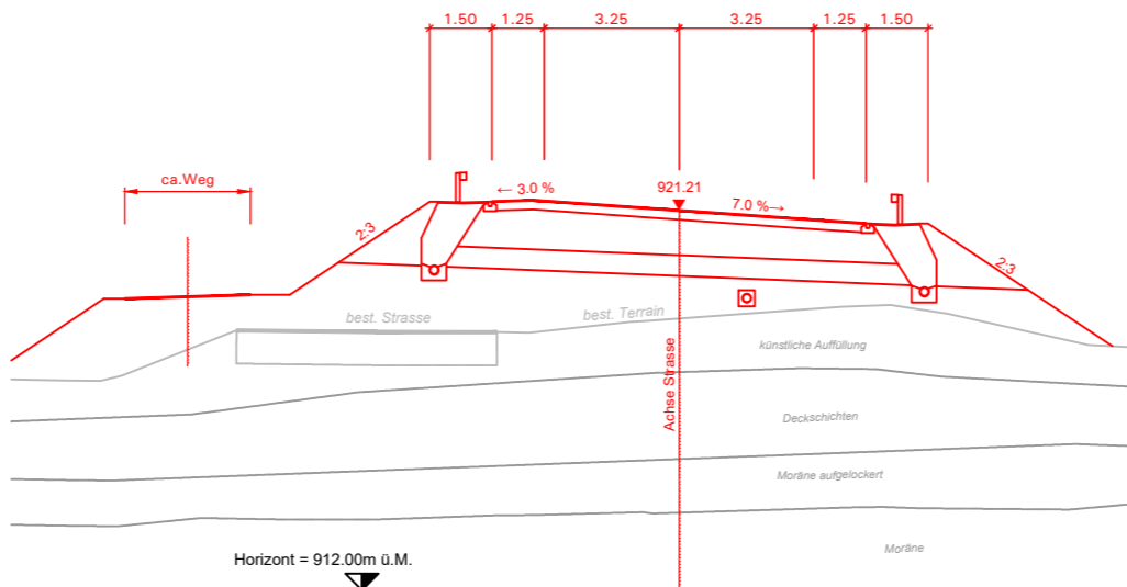
Schnitt 2-2
