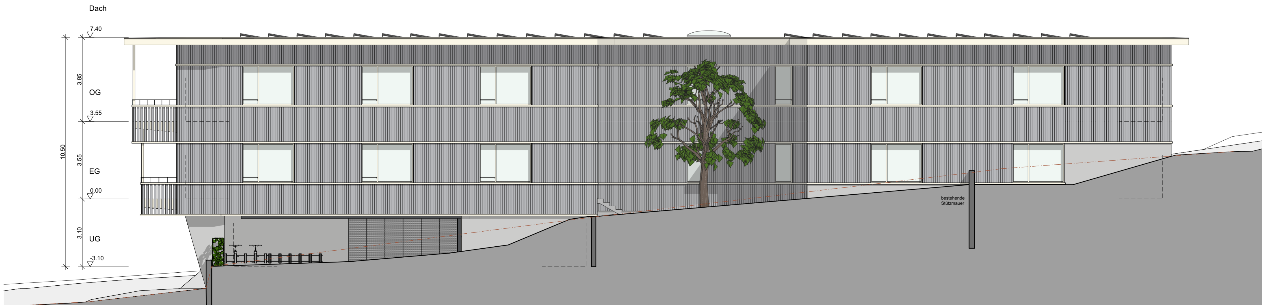
Ansicht West
