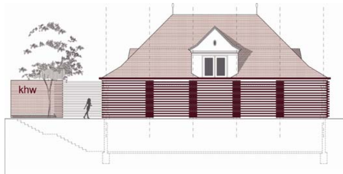
Westfassade Projektskizze Viola der Kleinviehmarkthalle (Quelle: zVg Stadt Wil)
