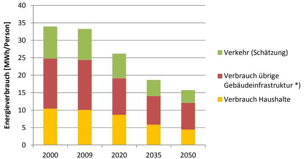
Abbildung 16: Energieverbrauchsszenario „Neue Energiepolitik“ bis 2050 für Kanton Glarus exkl. Prozessenergie von Grossverbrauchern, Daten aus nationalem Szenario umgelegt auf den Kanton Glarus (eigene Berechnung)
