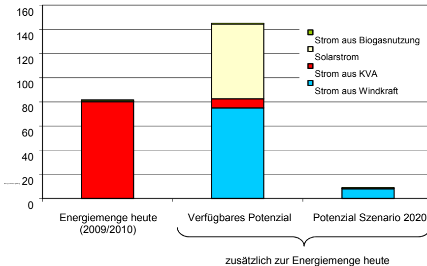
Abbildung 18: Potenzial für zusätzliche Stromproduktion ohne Wasserkraft im Vergleich zu heute
