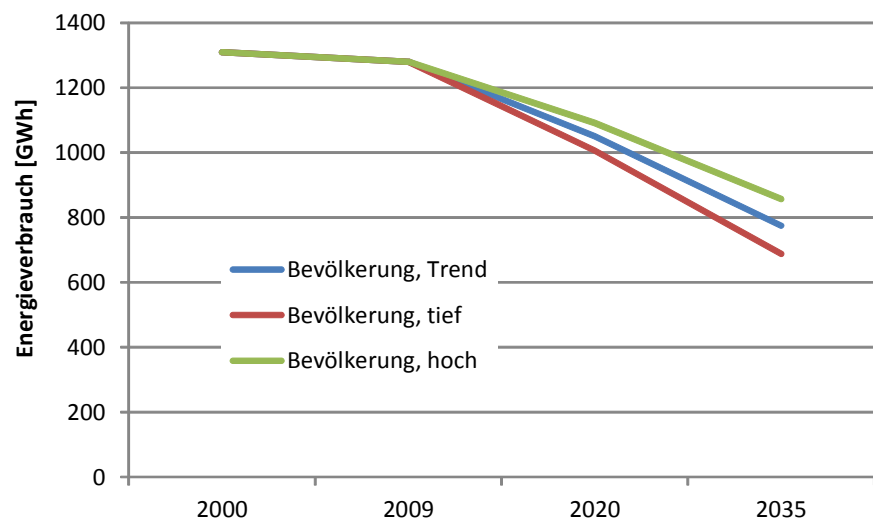
Abbildung 13: Energieverbrauchsszenario „Neue Energiepolitik“ bis 2050 für Kanton Glarus Daten aus nat. Szenario umgelegt auf den Kanton Glarus (eigene Berechnung)
