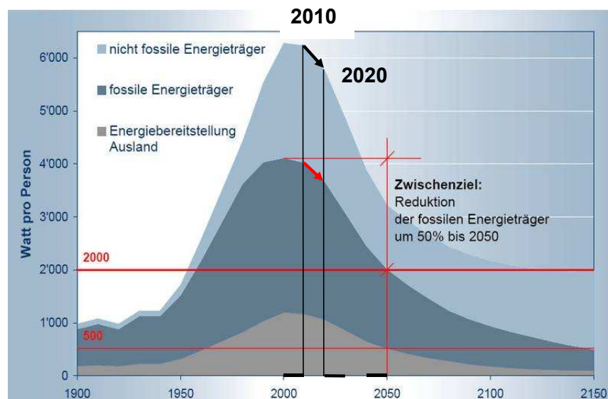
Abbildung 17: Zielpfad der 2000-Watt-Gesellschaft; Quelle: Novatlantis
