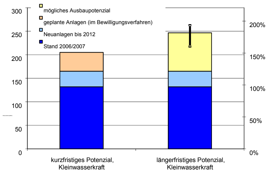
Abbildung 19: Potenzial für zusätzliche Stromproduktion aus Kleinwasserkraftwerken im Vergleich zu heute
