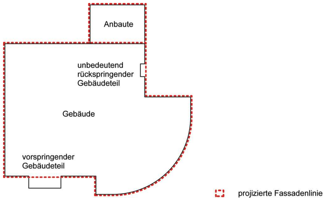
Figur 4: Projizierte Fassadenlinie
