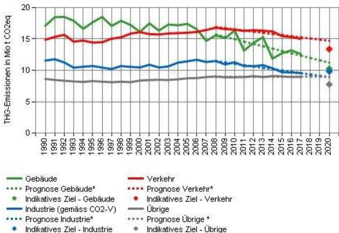
Abbildung 4: Sektorziele gemäss CO 2 -Verordnung, Entwicklung und Prognose für 2020
