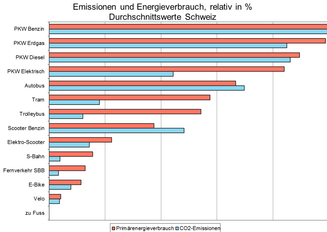
Abbildung 2: Emissionen und Primärenergieverbrauch von Verkehrsmitteln (Schweiz, 2016)
