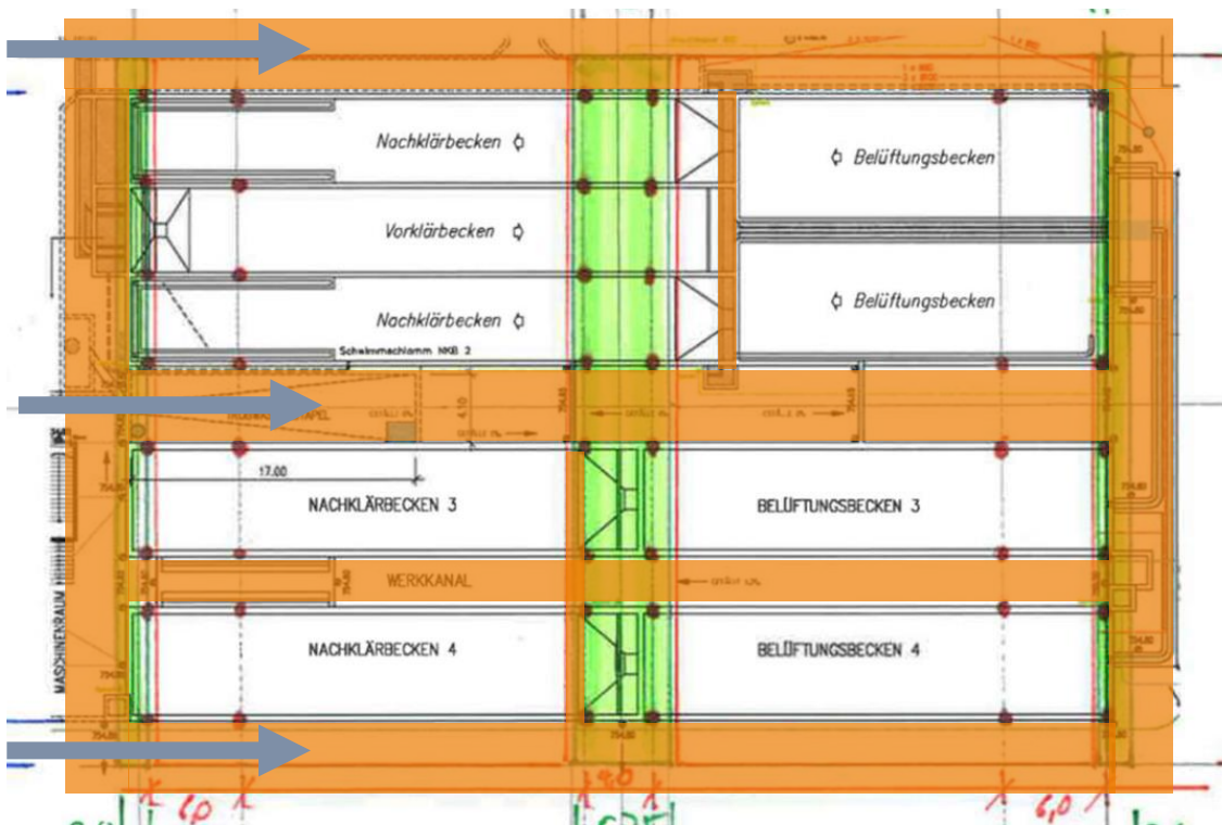
Abbildung 1: Die Positionierung der Abstützpunkte wurde während der Vorstudie statisch abgeklärt. Sie ist durchgehend auf den Beckenkronen möglich, es sind keine externen Fundamente notwendig. Die heutige Zufahrt ist weiterhin gewährleistet (orange Flächen). Die blauen Pfeile zeigen die Zufahrt in die ARA für LKWs.
