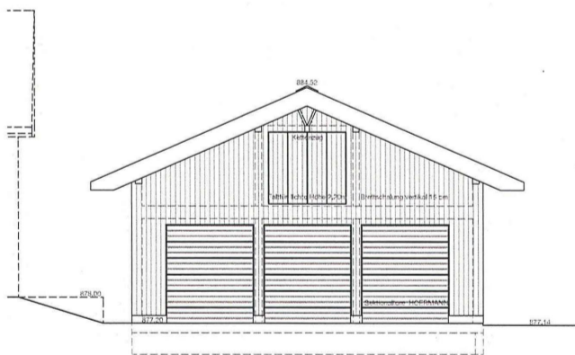
Ansicht Ökonomiegebäude von Osten
