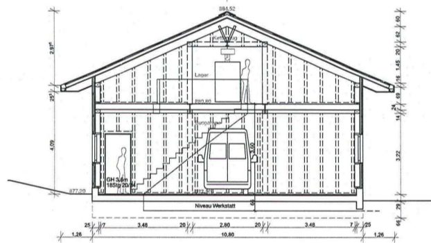
Querschnitt
