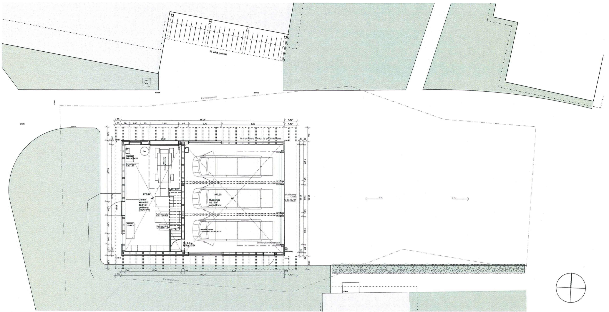
Situation Erdgeschoss Ökonomiegebäude
