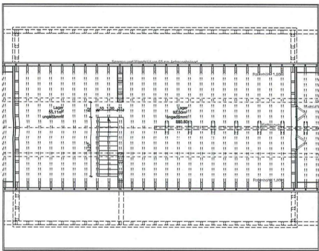
Dachgeschoss Ökonomiegebäude
