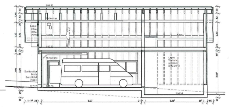
Längsschnitt
