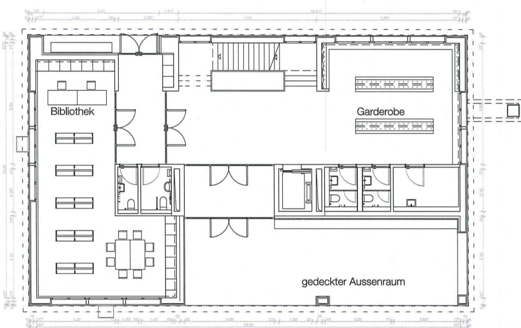
Erdgeschoss
