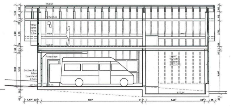
Längsschnitt
