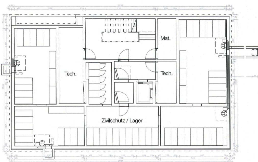
Untergeschoss
