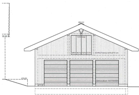
Ansicht Ökonomiegebäude von Osten
