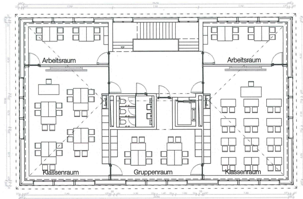
Dachgeschoss
