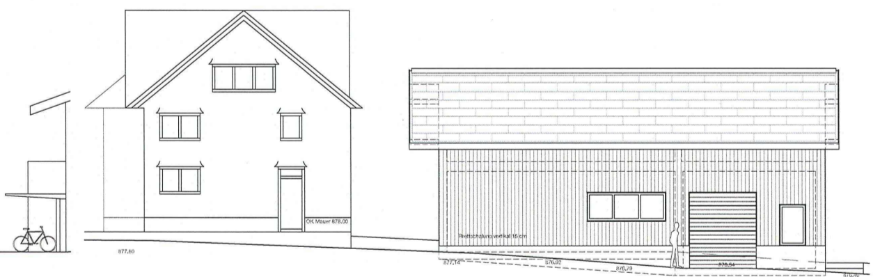
Ansicht Ökonomiegebäude von Norden
