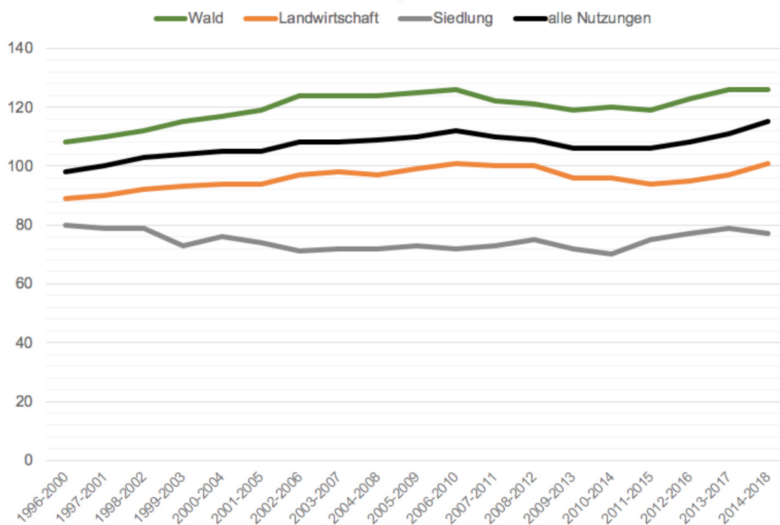
Abbildung 4: Die gleitenden 5 Jahres-Mittelwerte des Kessler-Index im Beobachtungszeitraum 1996 bis 2018 im ganzen Kanton Aargau. Er liegt 2018 für die Nutzungen Wald und Landwirtschaft beim höchsten Wert, welcher in der Zeitreihe seit 1996 ermittelt wurde.
