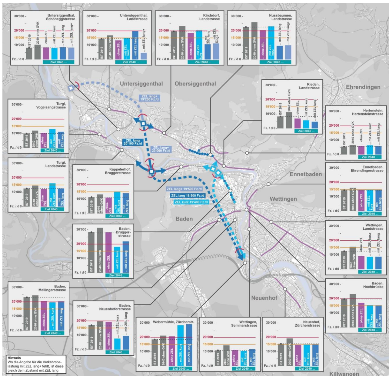
Abbildung 78: Tagesverkehrsbelastungen MIV (DWV) für GVK 2040 ohne bzw. mit ZEL im Vergleich zu Ist 2019 und Trend 2040
