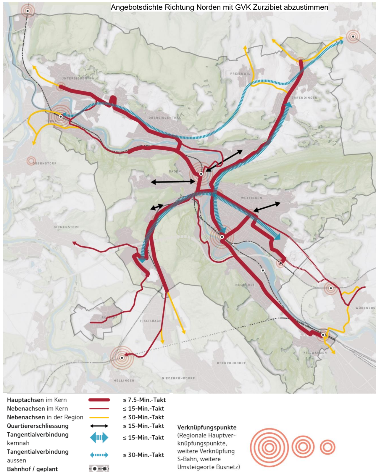
Abbildung 29: Grobkonzept Busnetz 2040
