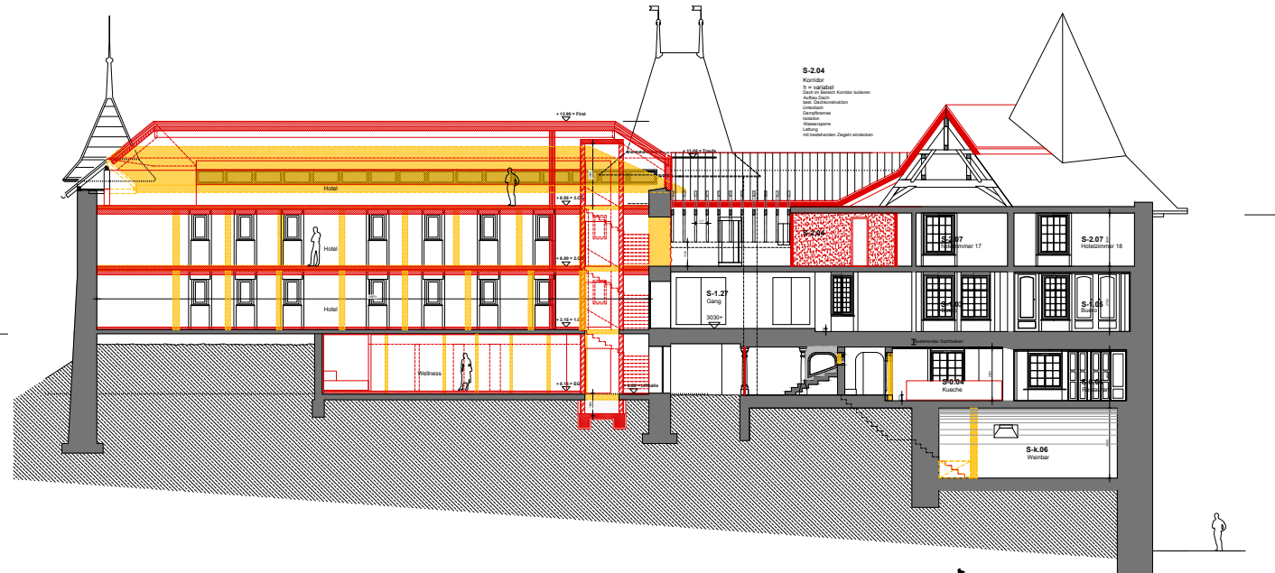
Längsschnitt D-D
