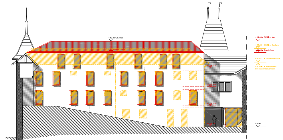
Hofansicht (West)
