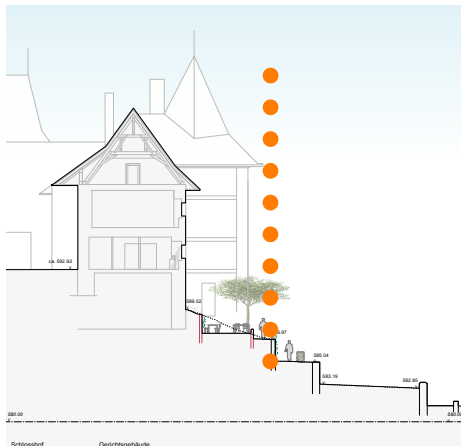
Schnitt A-A 1:200
