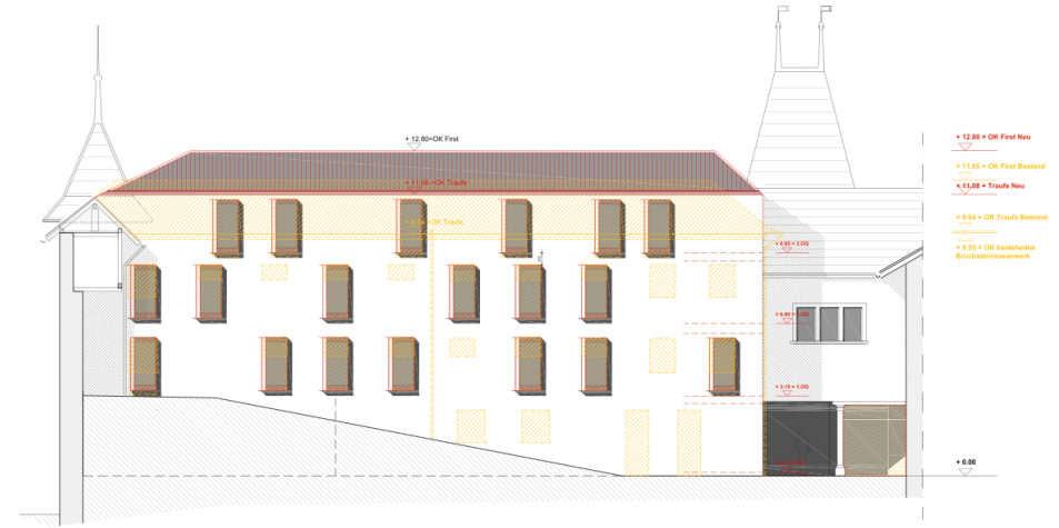
Hofansicht (West)
