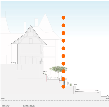
Schnitt A-A 1:200
