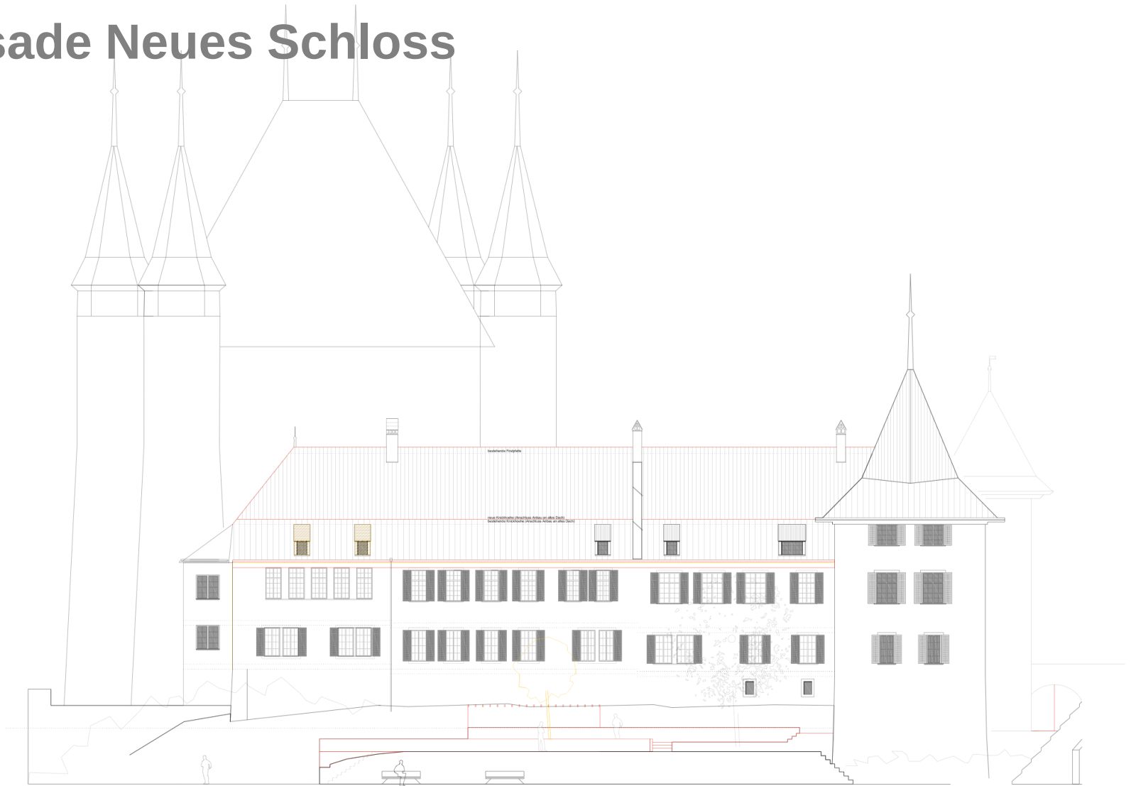
Aussenansicht (Süd)
