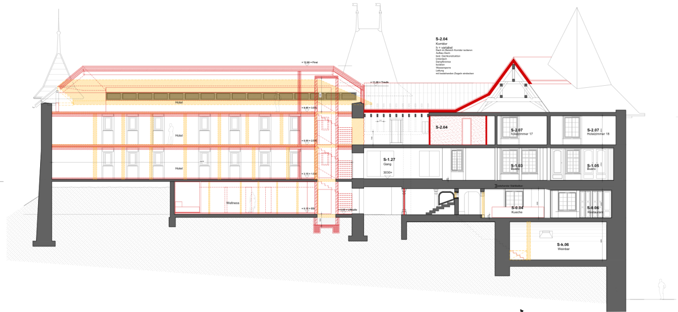
Längsschnitt D-D
