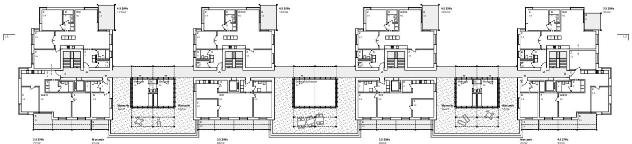
Abb. 18: 4. Vollgeschoss
