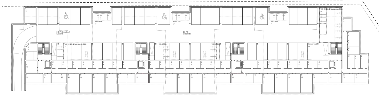
Abb. 16: Untergeschoss
