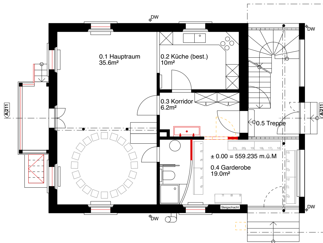
Erdgeschoss
