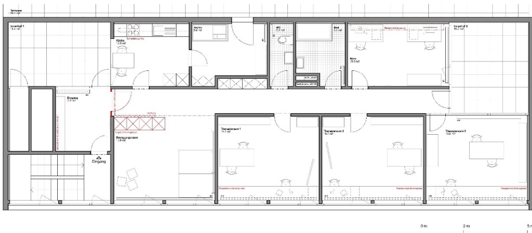
Grundriss
