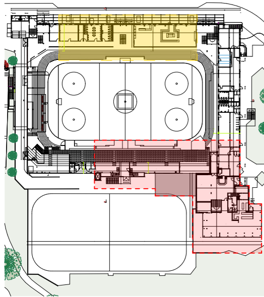
PHASE 02A Travaux Aile Ouest Restaurant Démolition Aile Est
