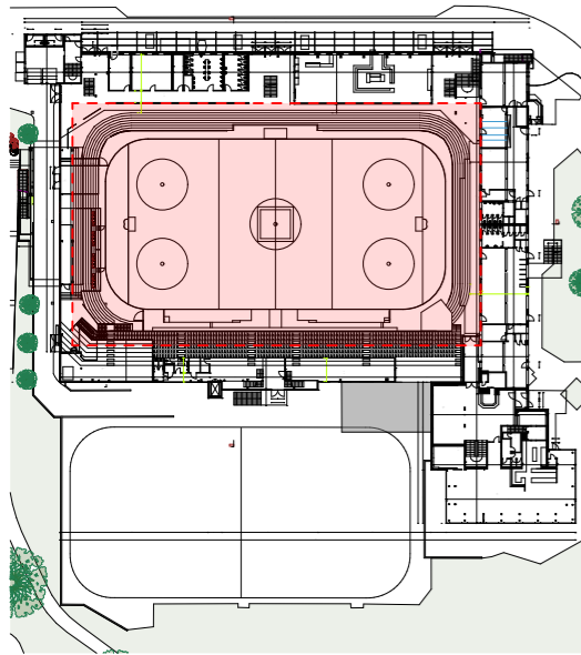
PHASE 03 Démolition et travaux Toiture
