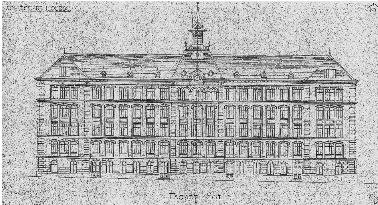
Façade Sud
