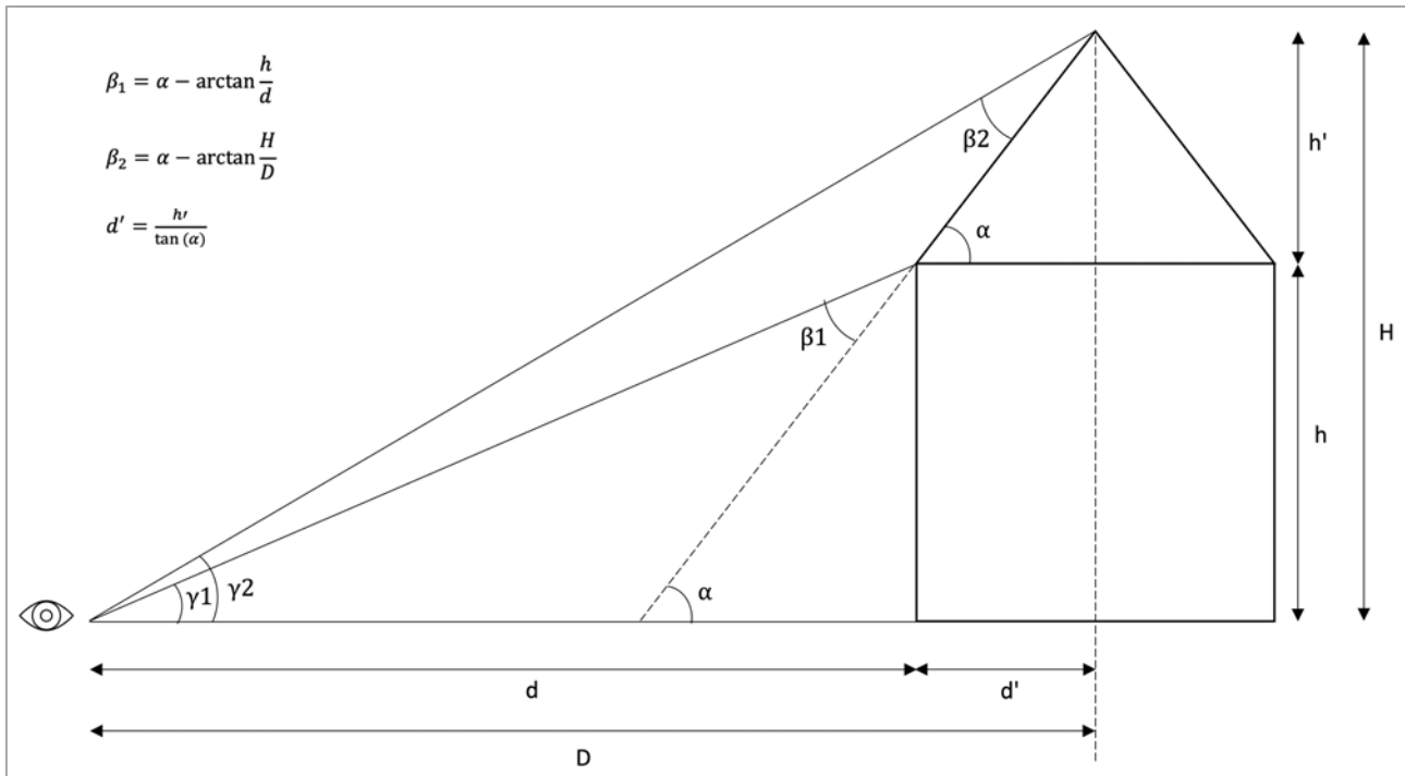
Figure 28 : Angles de vue de la rue sur la toiture et les panneaux solaires
