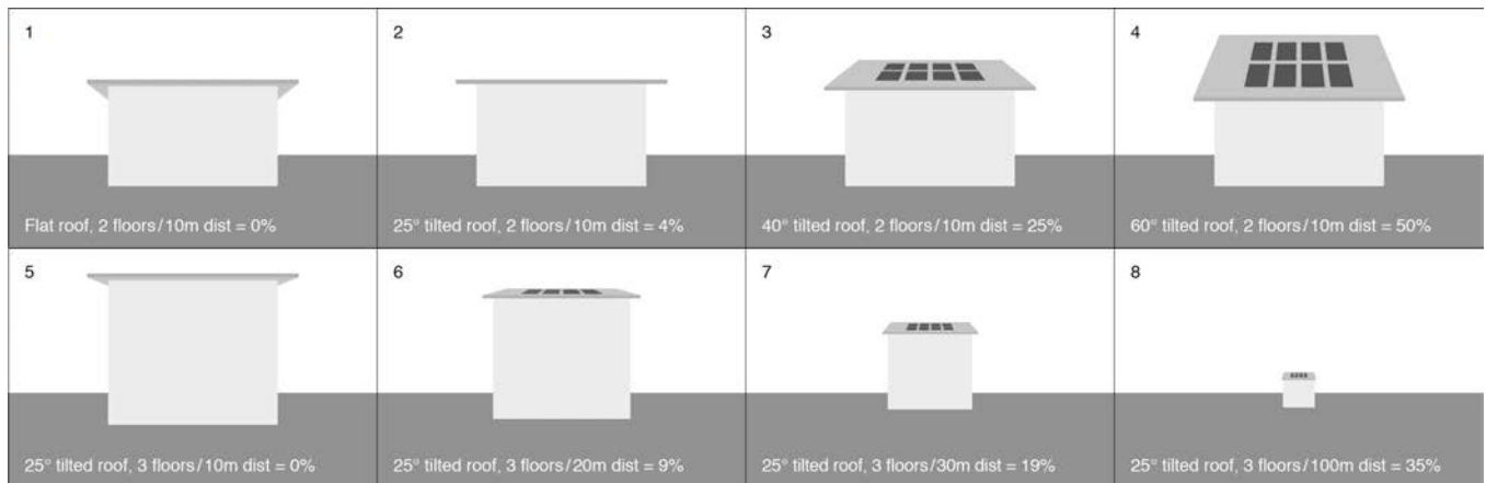
Figure 29 : Simulation de l'impact visuel des distances d'observation pour un bâtiment de 3 étages avec un toit en pente (Crédits EPFL/LESO-PB)
