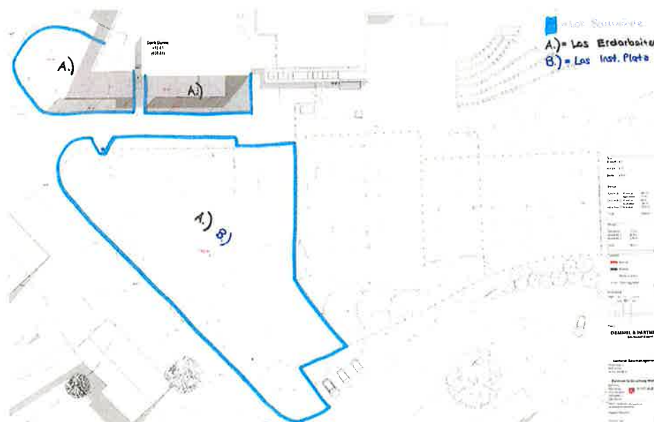
Abbildung Lageplan, Losaufteilung (A: Los Erdarbeiten, B: Los Installationsplatz, C: Los Bauwände)
