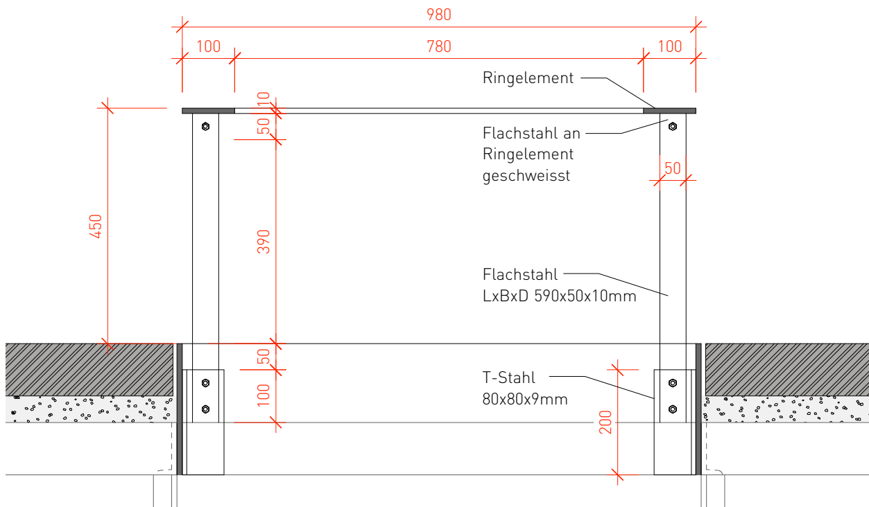
Schnitt M 1:10
