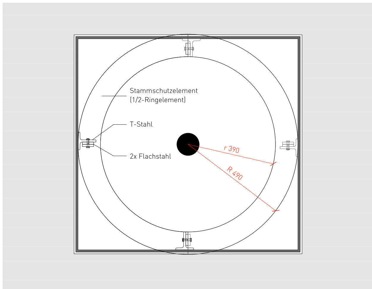
Grundriss M 1:10
