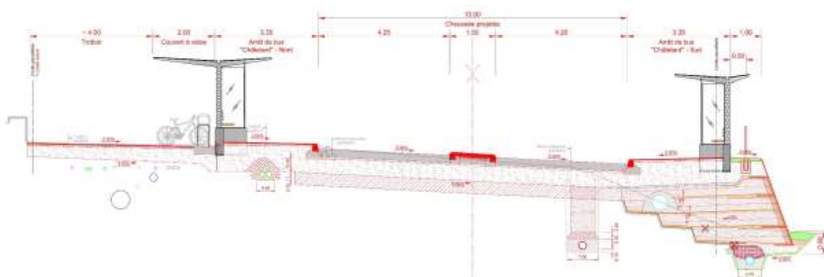
Figure 8: coupe-type du projet du carrefour du Châtelard
