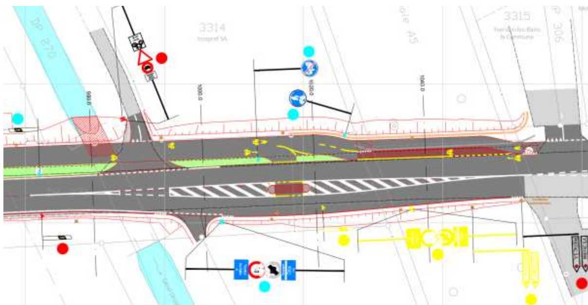
Figure 5: extrait de situation du tronçon sur Yverdon-les-Bains dont la porte d'entrée vers le profil 1000.0
