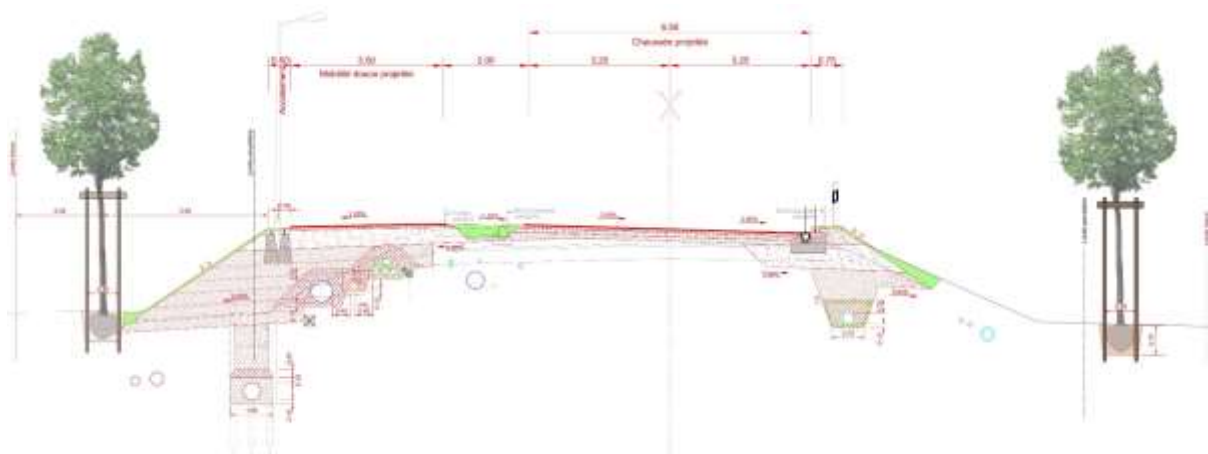
Figure 6: coupe-type du tronçon sur Yverdon-les-Bains
