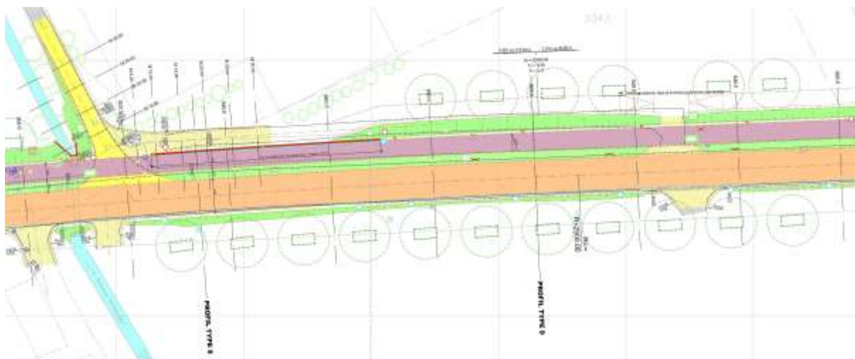
Figure 4 : extrait de situation du tronçon sur Yverdon-les-Bains dont la section type
