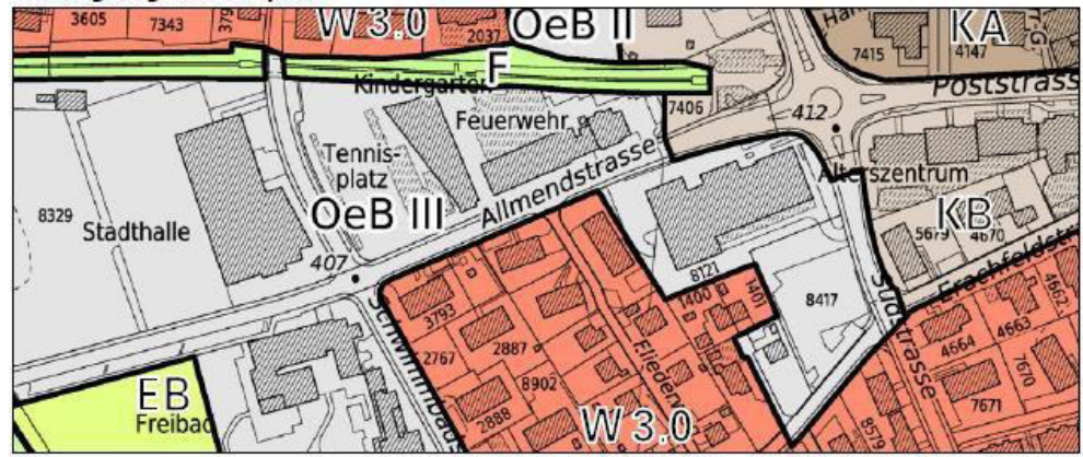
Rechtsgültiger Zonenplan
