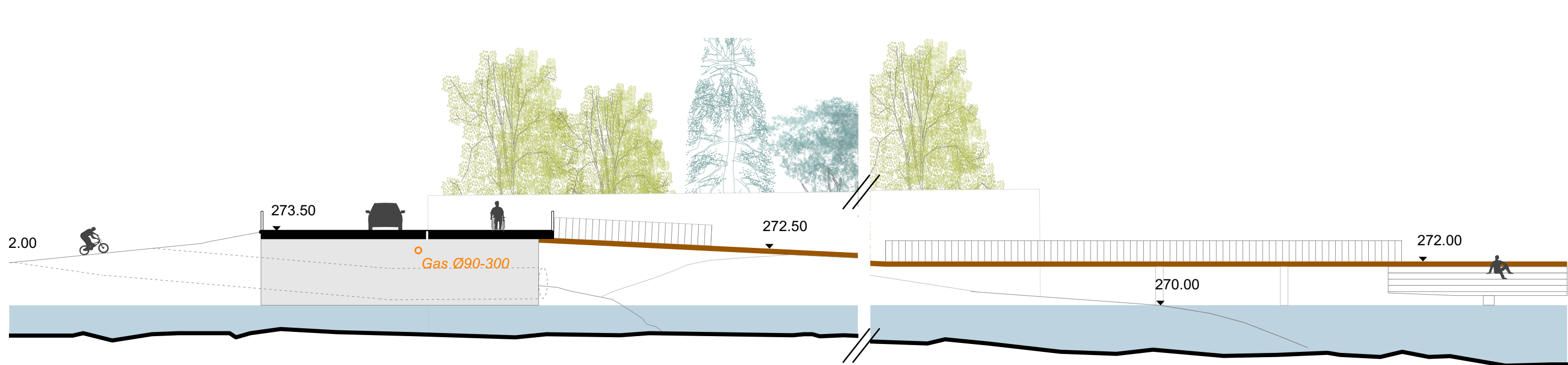
Passeggiata sulla passerella del Lido del Laveggio - Sezione C-C' 1:200
