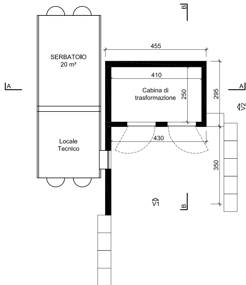
PIANTA
