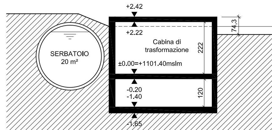
SEZIONE A-A
