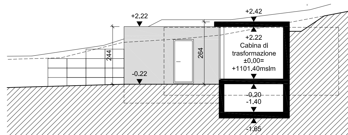
SEZIONE B-B
