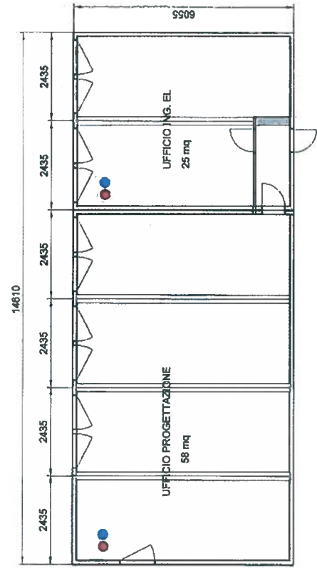
BLOCCO 2 SOPRA BLOCCO 1 con scala esterna
