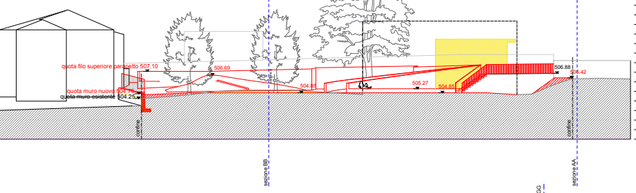
SEZIONE FF
