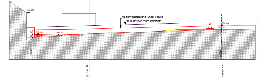
SEZIONE EE
