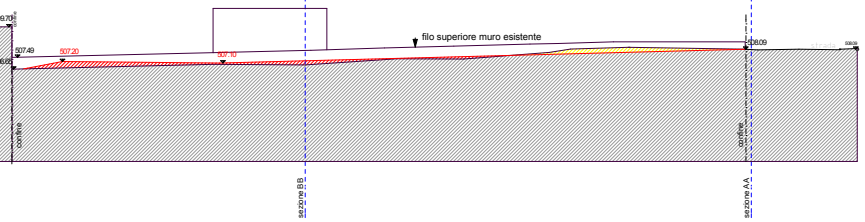
SEZIONE DD lungo muro esistente parcheggio confinante fondo 1202
