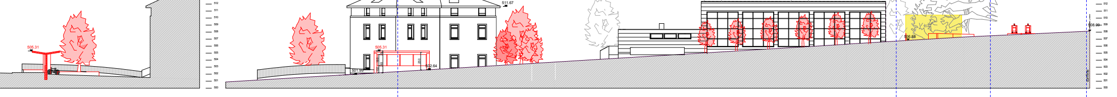
SEZIONE GG
