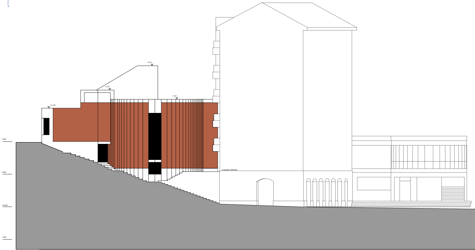
FACCIATA EST
