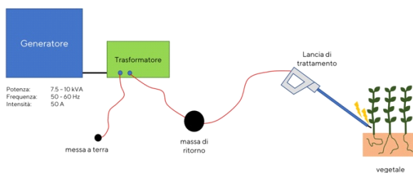
Elettrodiserbo - schema semplificato del funzionamento
