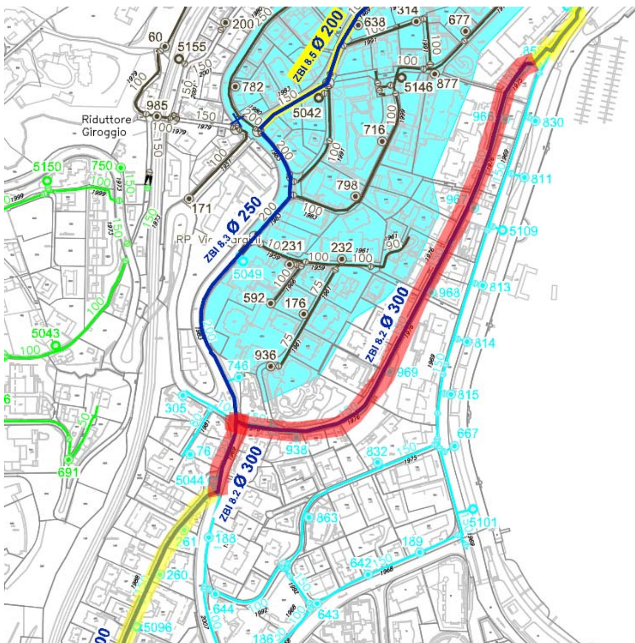
Figura 1 Collegamento serbatoio Via Mazzini – Via Cassarinetta a Loreto (vedi tratta in colore rosso ca. 700 m DN 300 mm)
