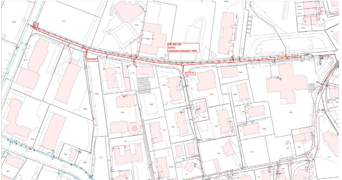
Figura 3 Via Maraini a Pregassona (vedi tratta in colore rosso 350 m DN 200 mm)
