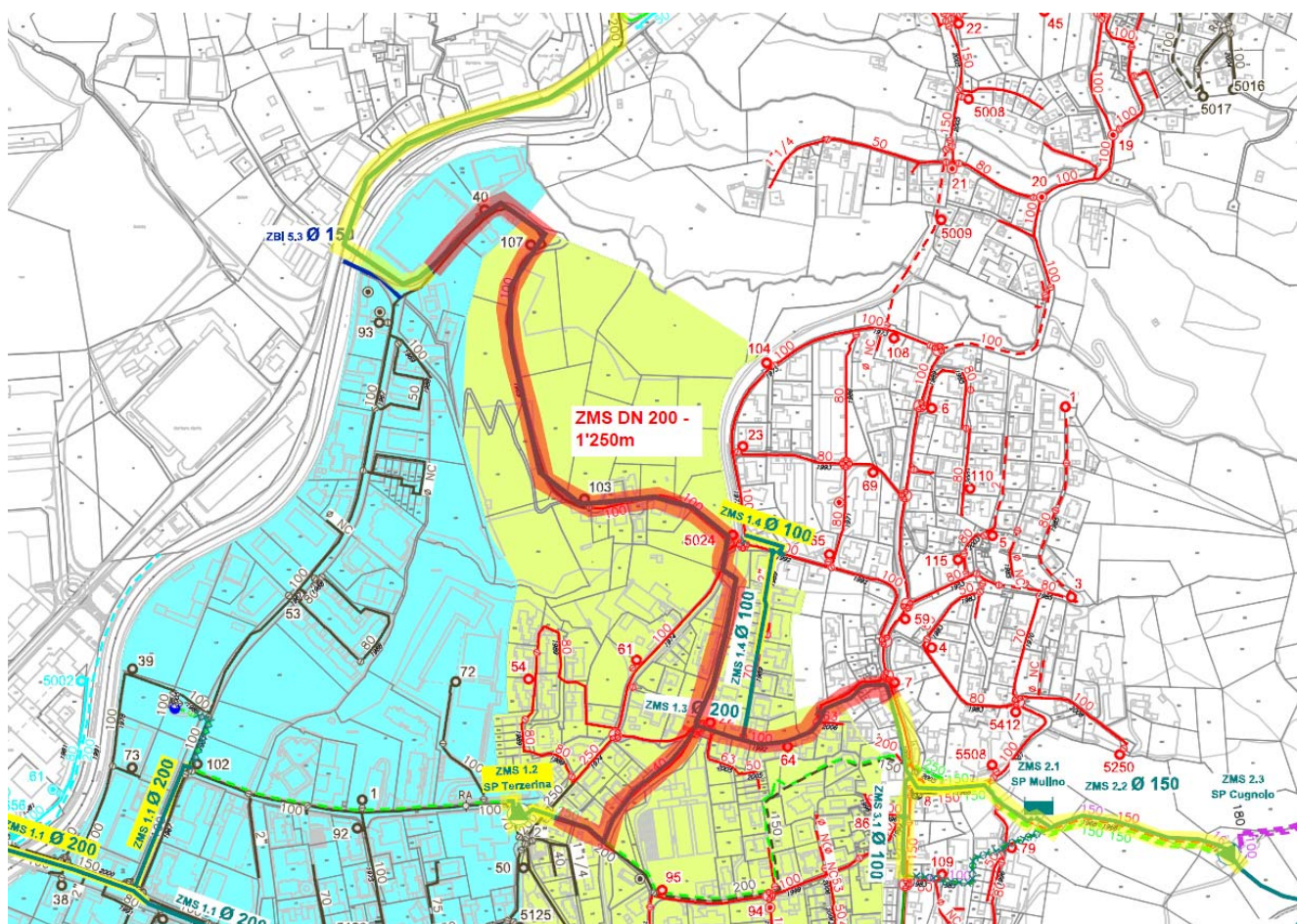
Figura 2 Collegamento Ponte di Valle - Serbatoio Mulino - Stazione pompe Terzerina a Pregassona (vedi colore rosso 1'250 DN 200 mm)
