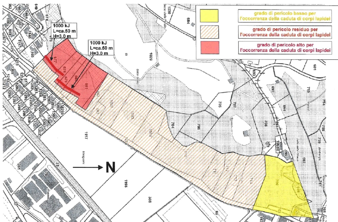
Intervento via delle Scuole - Carta dei pericoli post-intervento
