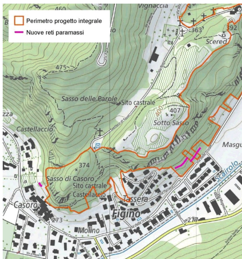
Perimetro progetto integrale e ubicazione interventi di premunizione
