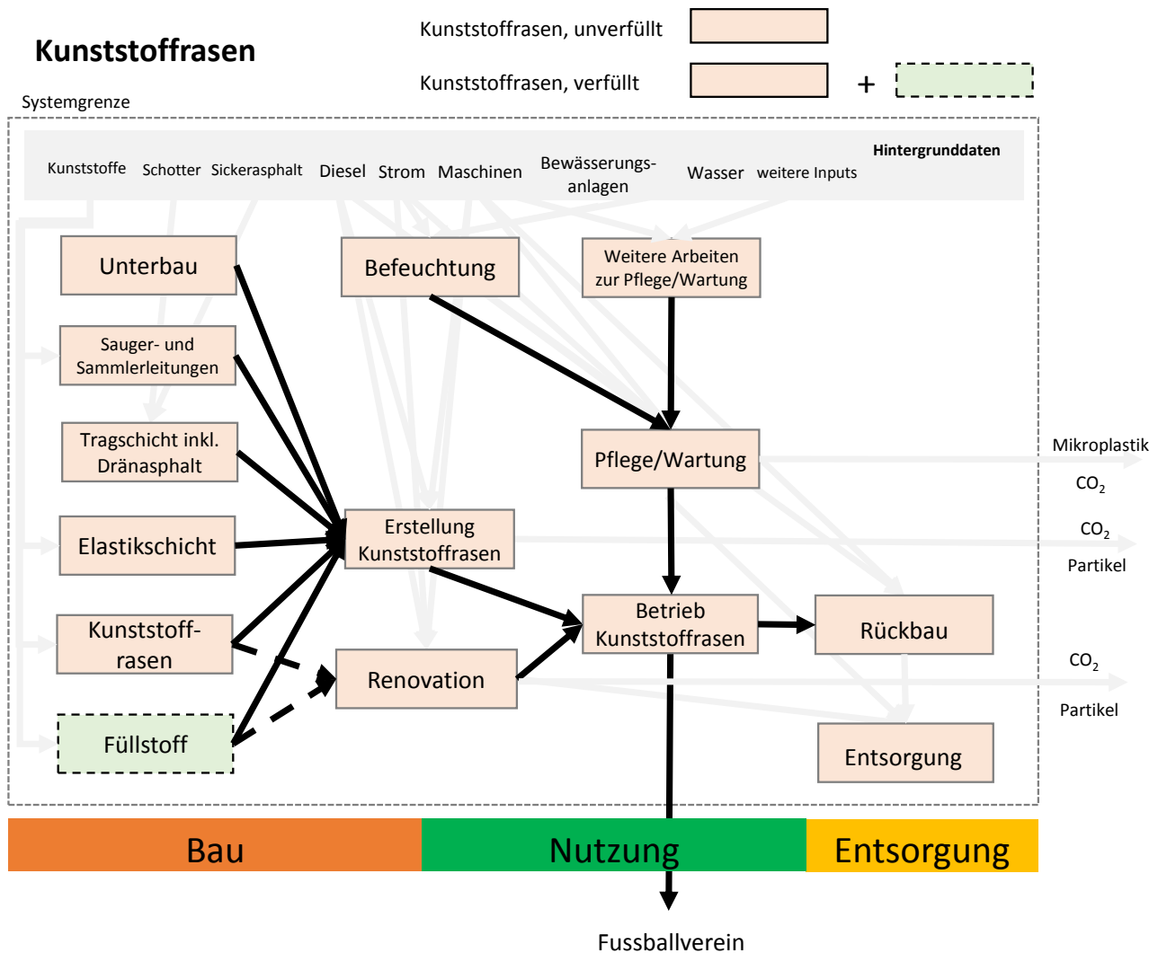
Abbildung 1: Systembild des Kunststoffrasensportfeldes. Orangegefärbte Prozesse sind bei allen Kunststoffrasen vorhanden, hellgrüngefärbte Prozesse sind nur bei den verfüllten Kunststoffrasen vorhanden.
