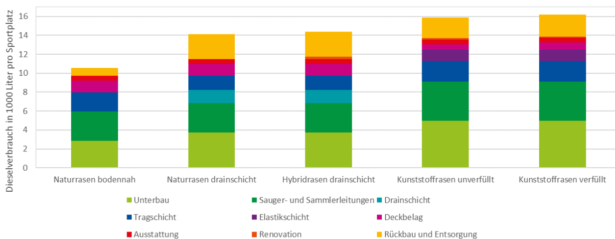
Abbildung 3: Dieserverbrauch in 1000 Liter dargestellt, welcher bei der Erstellung eines Rasensportfeldes anfällt. Die Dieserverbräuche sind anhand des Aufbaus unterteilt und nach Rasensportfeld gruppiert.
