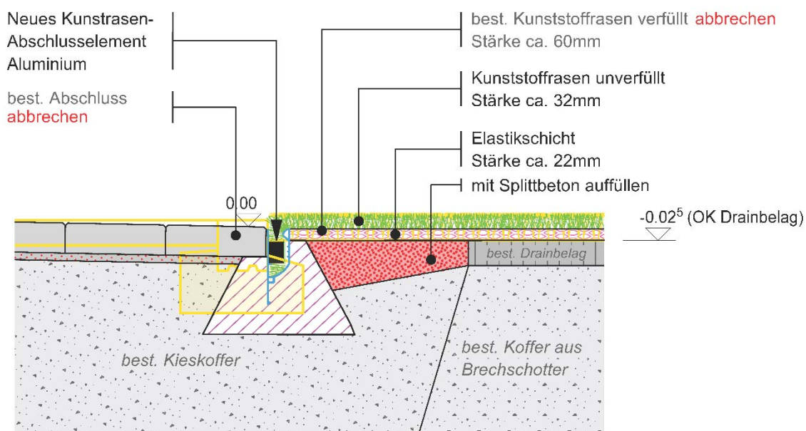
Abbildung 5: Details Kunstrasen unverfüllt, bhateam ingenieure ag
