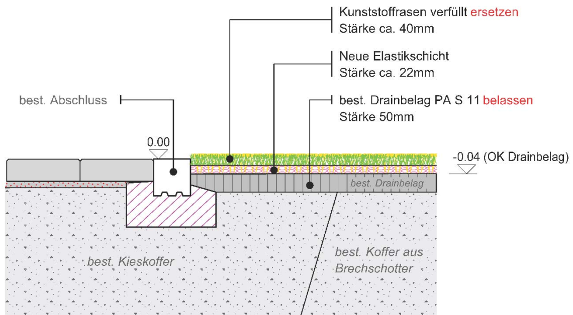
Abbildung 4: Details Kunstrasen verfllt, bhateam ingenieure ag
