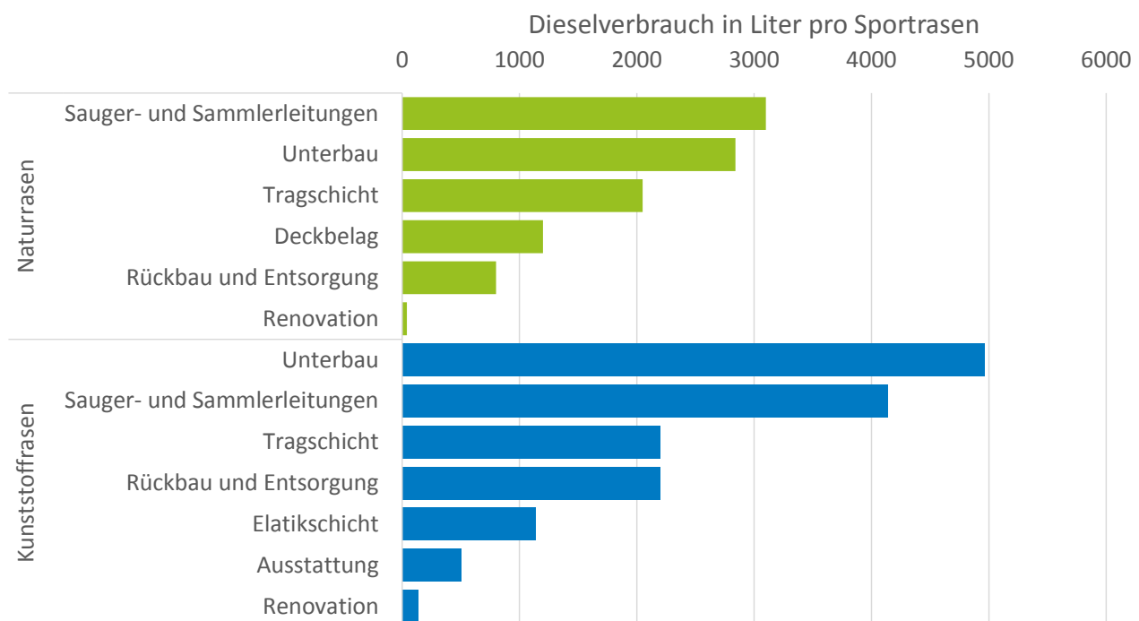
Abbildung 4: Dieserverbrauch pro Sportplatz und Pflegejahr. Die Pflege von Hybrid- und Naturrasen ist identisch und verursacht einen deutlich höheren Dieserverbrauch als die Pflege von Kunststoffrasen. Das Mähen, sowie das Aufnehmen beim Natur- und Hybridrasen sind dabei die grössten Faktoren.
