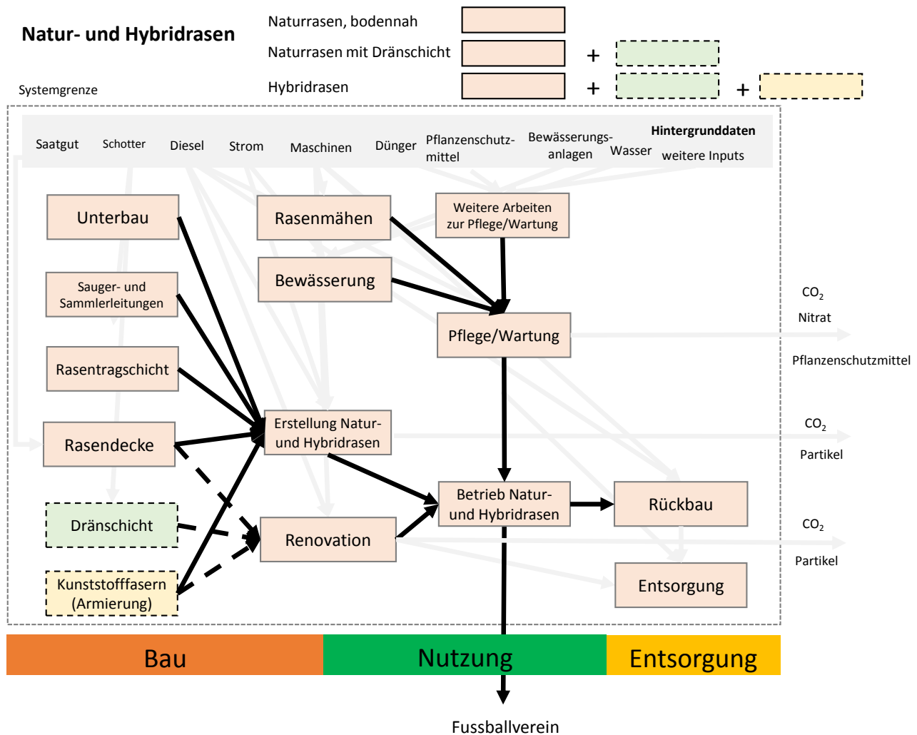
Abbildung 2: Systembild der Natur- und Hybridrasen. Orangegefärbte Prozesse sind bei allen Natur- und Hybridrasen vorhanden, hellgrüngefärbte nur bei den Naturrasen mit Dränschichtbauweise und den Hybridrasen, gelbgefärbte Prozesse sind nur bei den Hybridrasen vorhanden.
