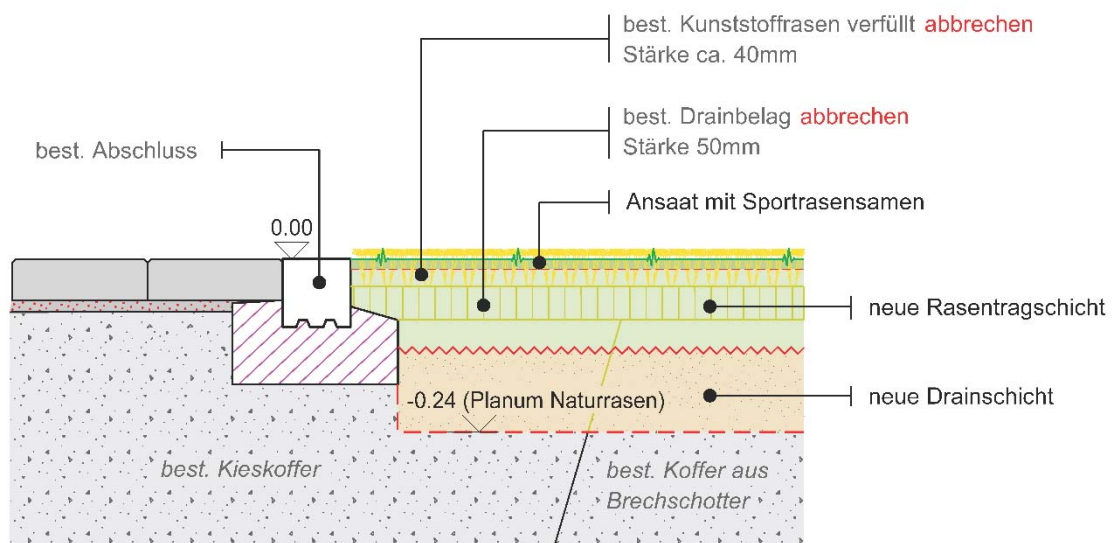
Abbildung 3: Details Naturrasenaufbau, bhateam ingenieure ag
