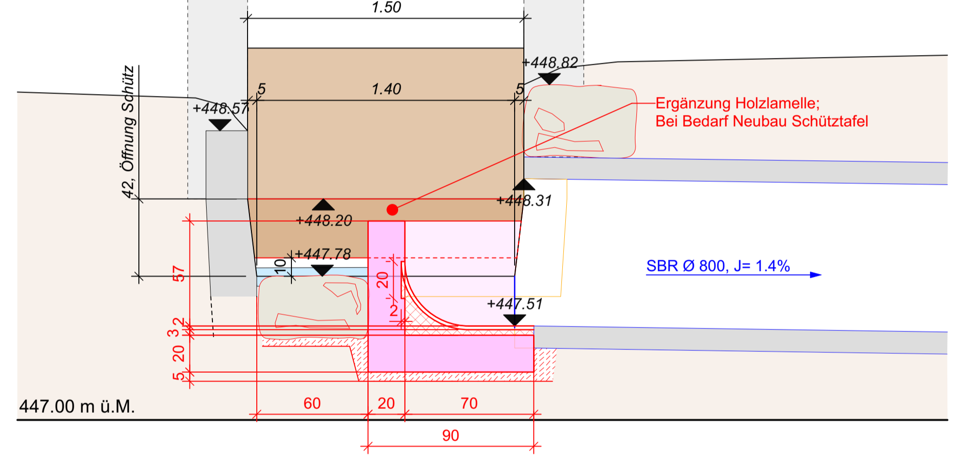
QP2 Schütz M 1:20
