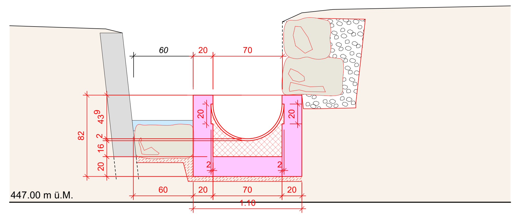
QP1 Überlauf, M 1:20
