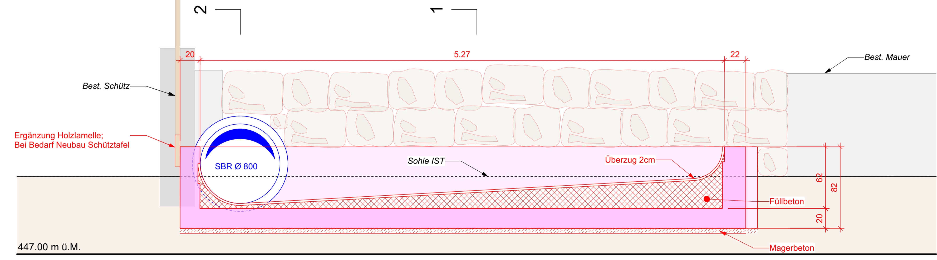
LP Überlauf und Schütz M 1:20
