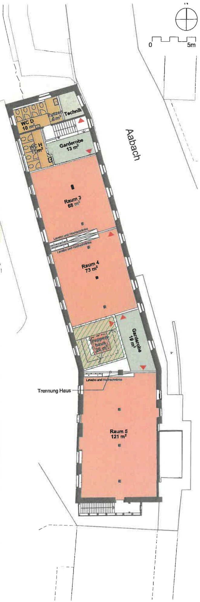
Grundriss Obergeschoss | Mst. 1:250
