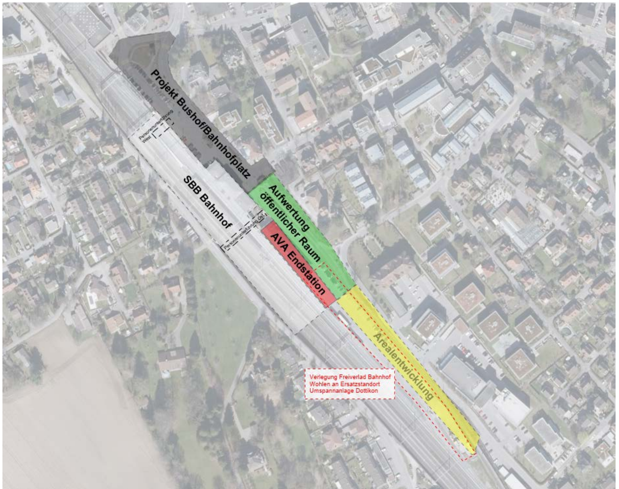
Abbildung: Übersicht Projektbestandteile ÖV Drehscheibe Bahnhof Wohlen
