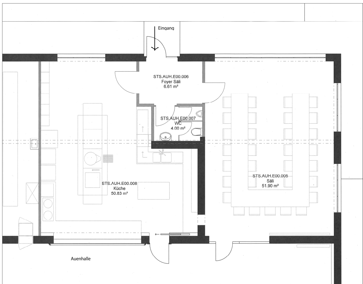
Grundriss EG Auenhalle: Säli und Küche
