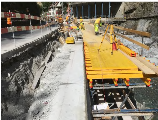
Schalung Kragtrottoir
