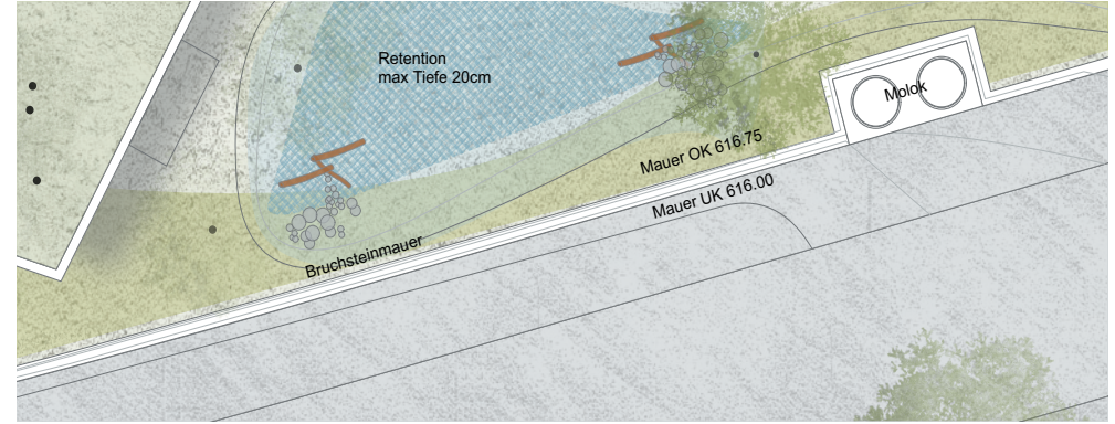
Bruchsteinmauer entlang der Cadonastrasse
