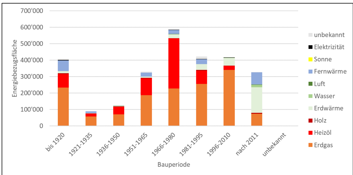
Abbildung 6: Zubau von Energiebezugsfläche aller Liegenschaften (nur Haushalte) nach Baujahr und der aktuell im GWR angegebenen Heizungsart (Quelle: Ecospeed Immo2023, Basis Gebäude und Wohnregister).
