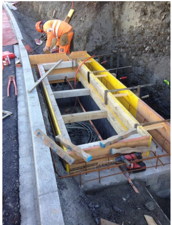
Schalung für Betonkranz EW-Schacht
