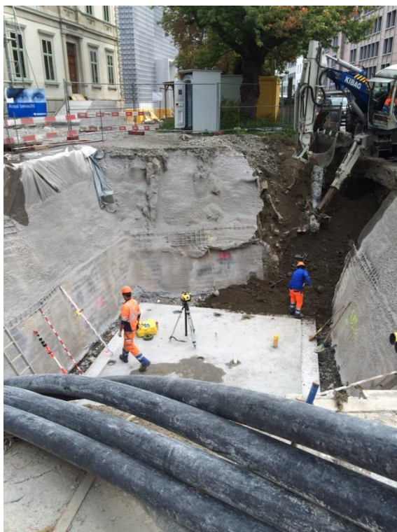
Bodenplatte und Innenleben der neuen unterirdischen Trafostation der IBC
