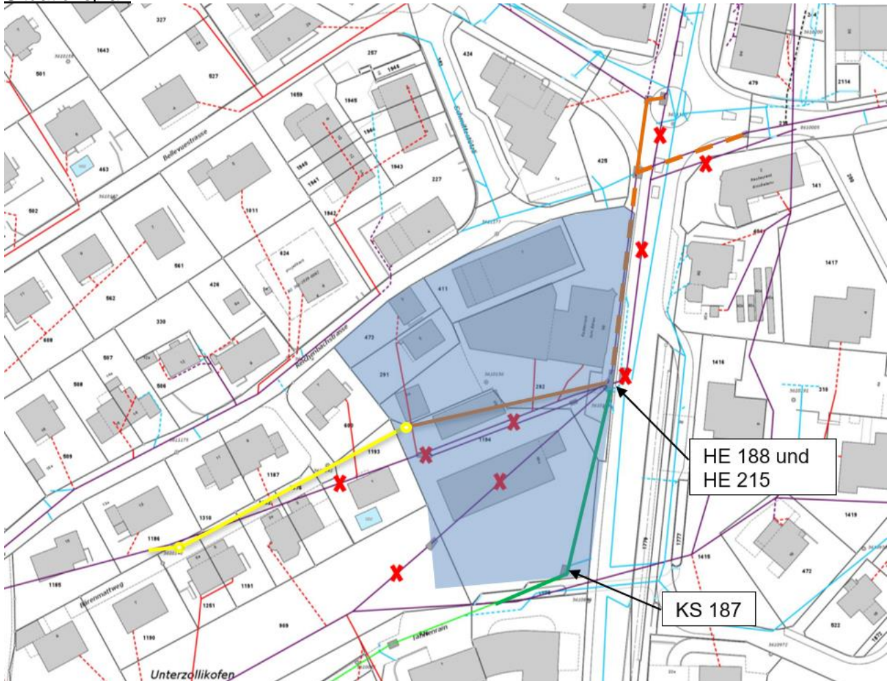
Abb. 1 Situationsplan: orange = Teilprojekt 1 Leitung Bärenareal und Kreisel gelb = Teilprojekt 2 Bärenmattweg grün = Teilprojekt 3 Entlastungsleitung blau = Perimeter Überbauung Bärenareal
