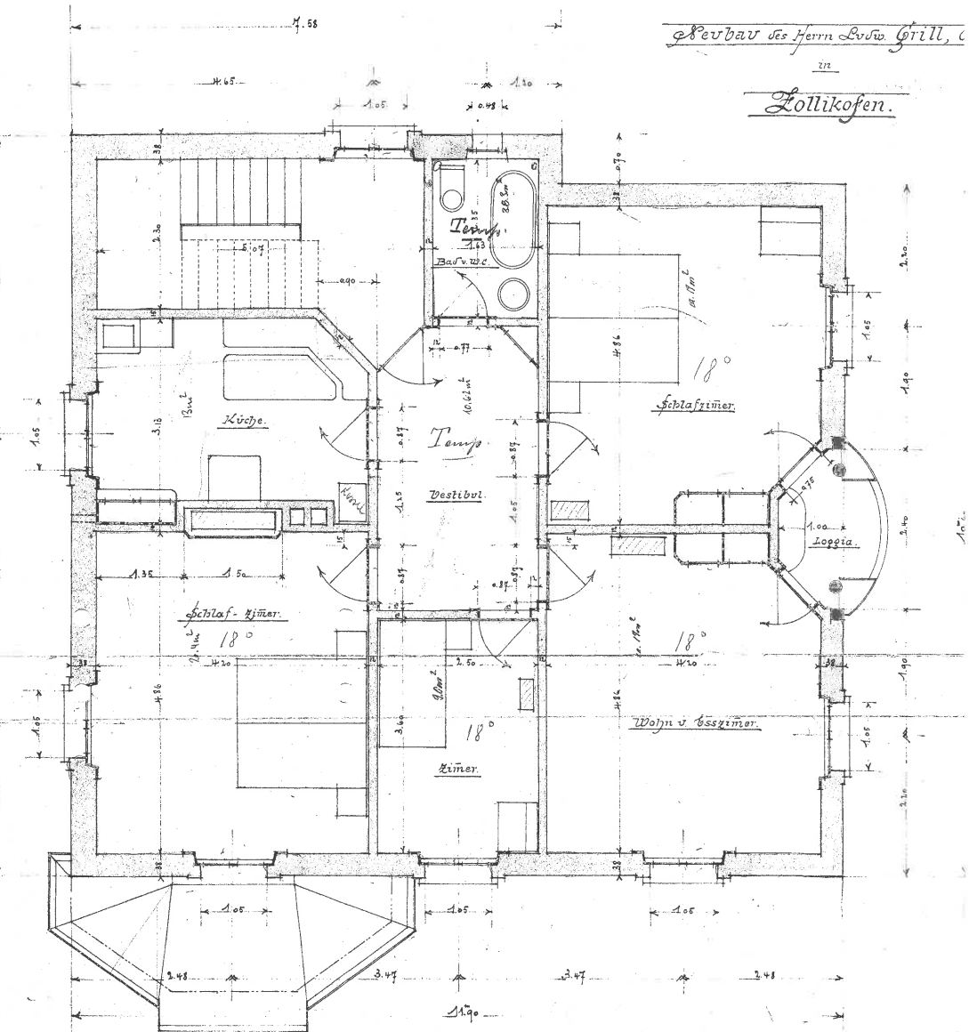
Grundriss d. I. Stock. 94.80
